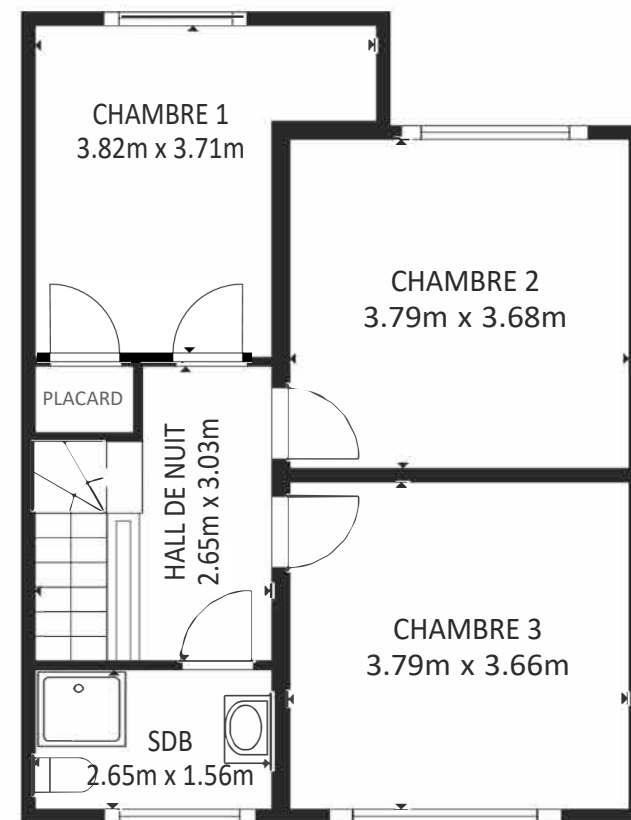
1er ETAGE
