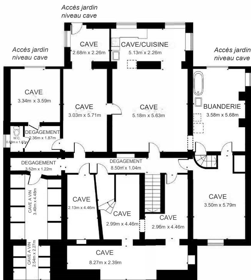
SOUS-SOL Surfaces intérieures brutes +/- 246 m 2
