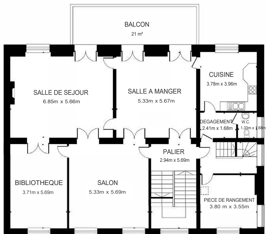
1er ETAGE Surfaces intérieures brutes +/-195.5 m 2
