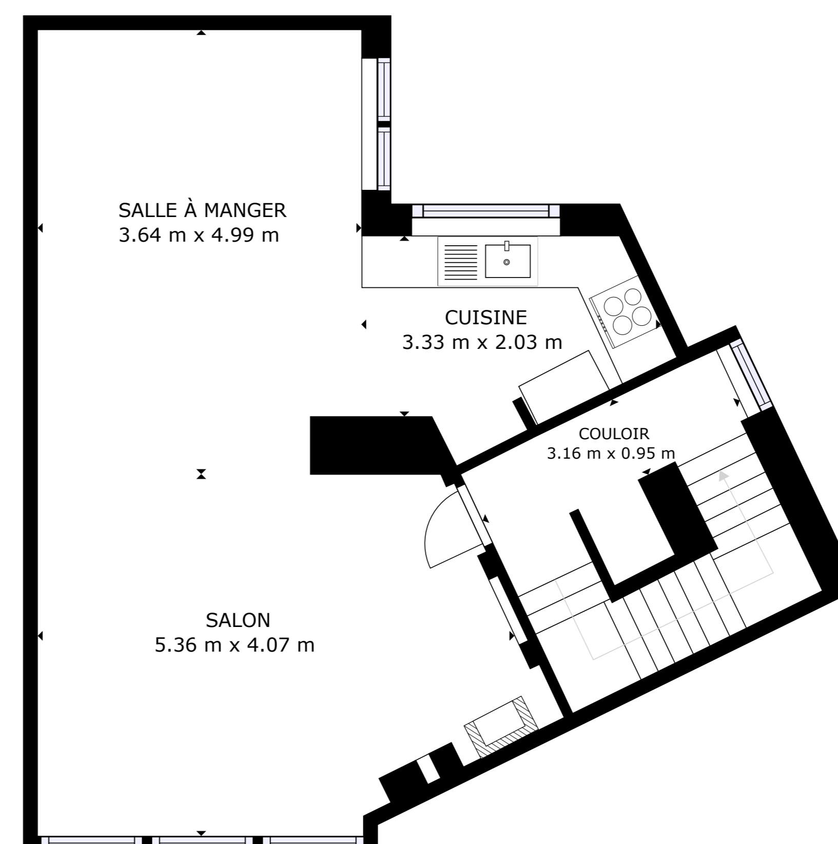
1ER ETAGE
