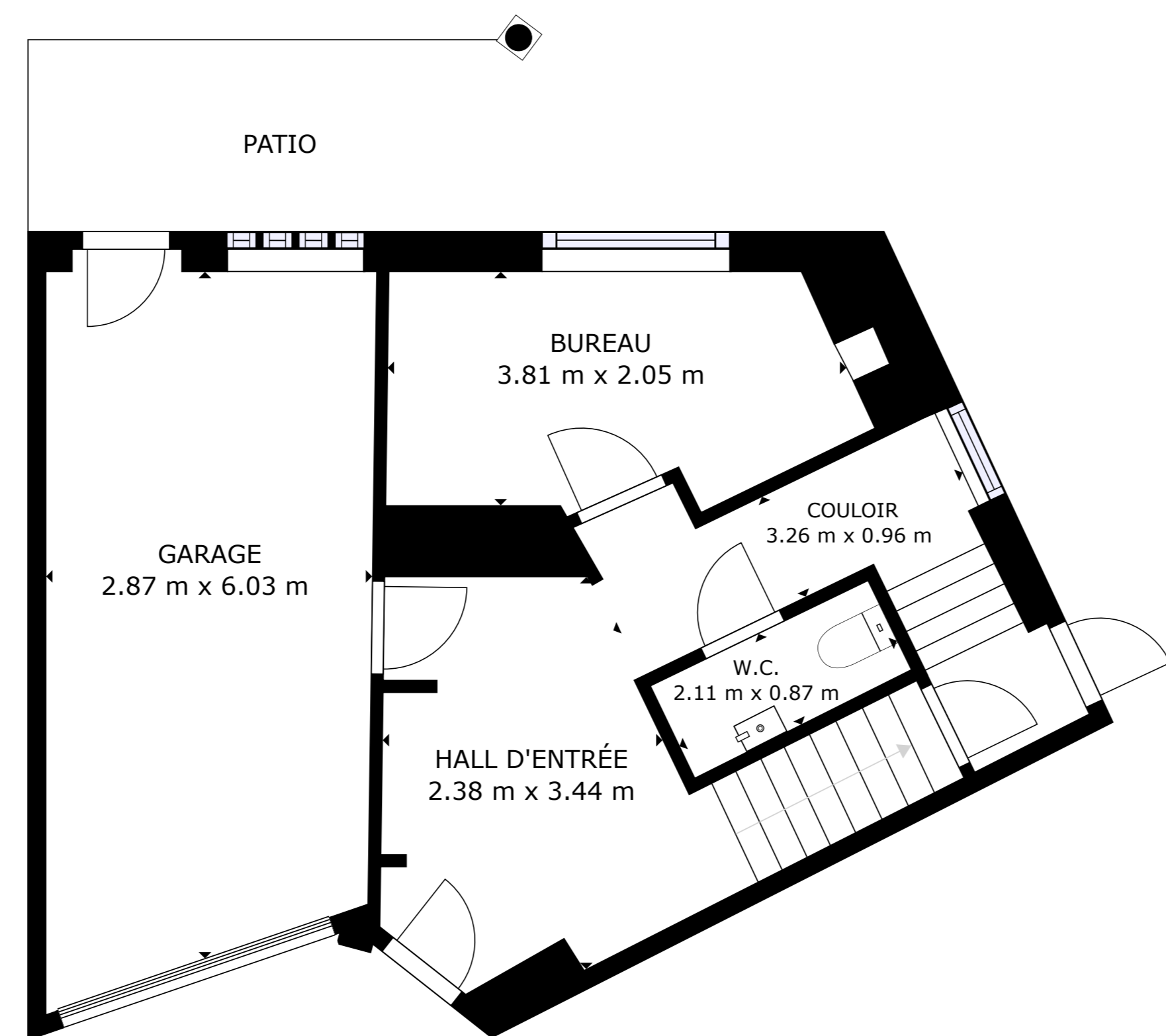
REZ-DE-CHAUSSEE
