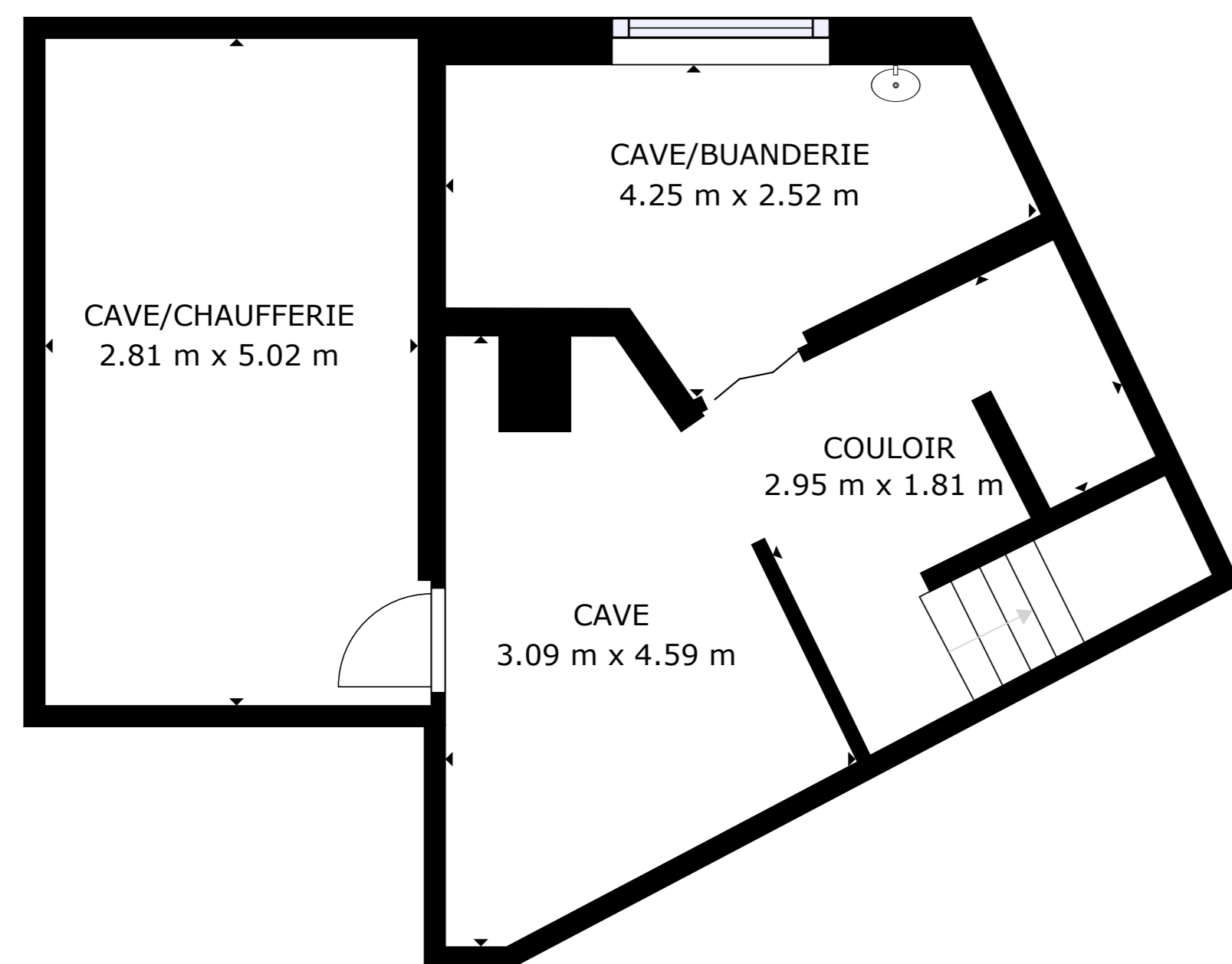
SOUS-SOL
