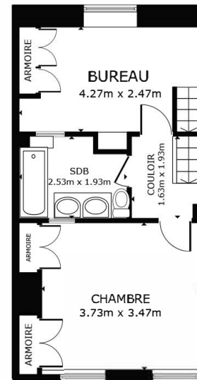
1er ETAGE
