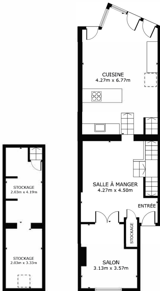
SOUS-SOL
