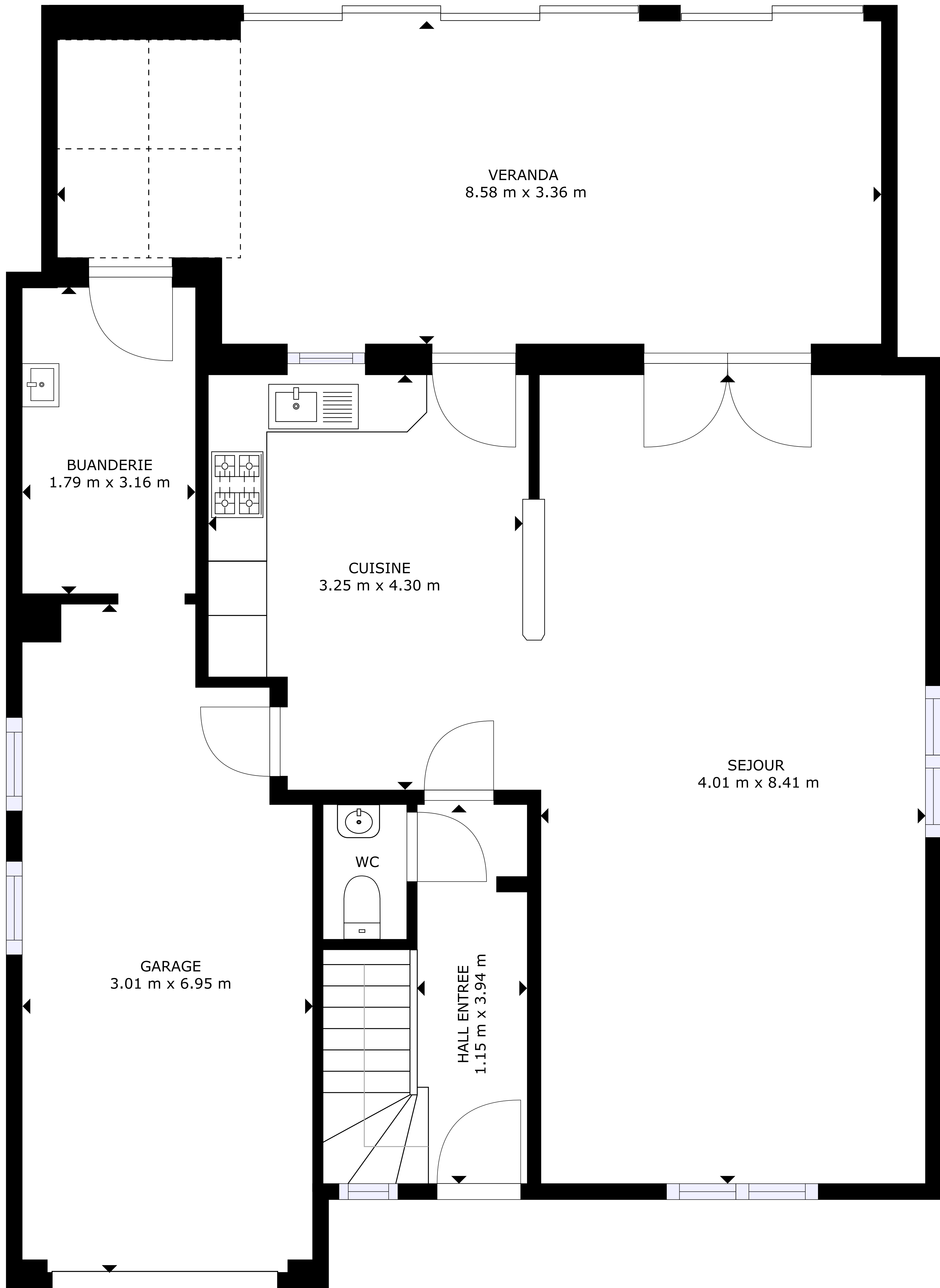
REZ-DE-CHAUSSEE
