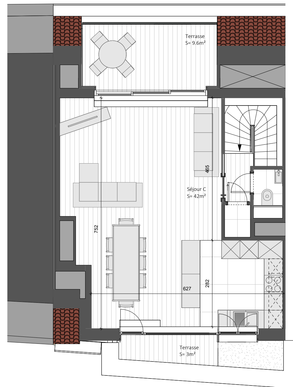
Troisième Etage
