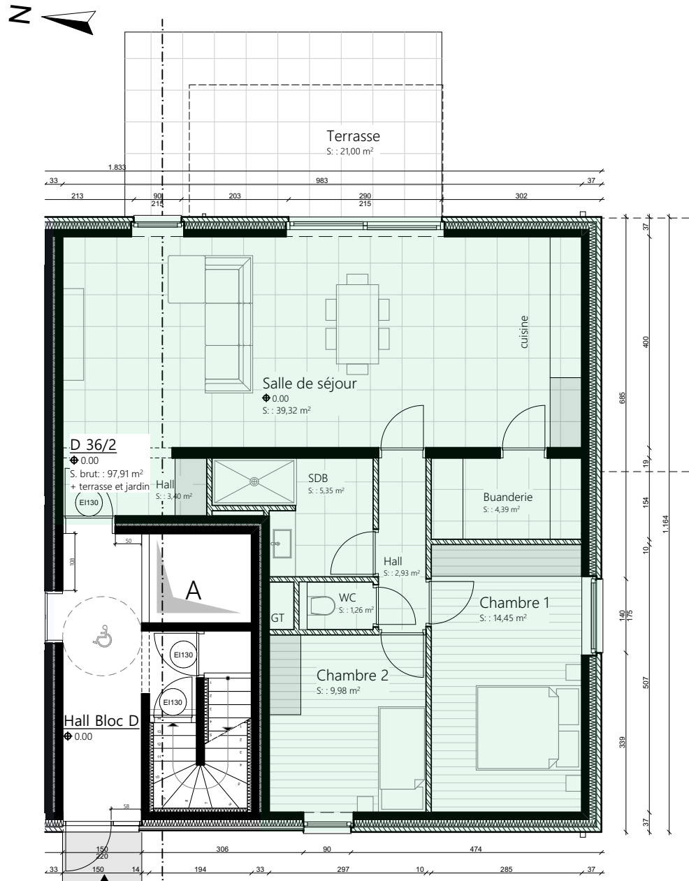
0. Rez-de-chaussée 1:100
