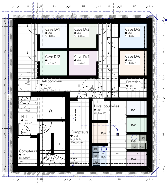
-1. Sous-sol 1:150
