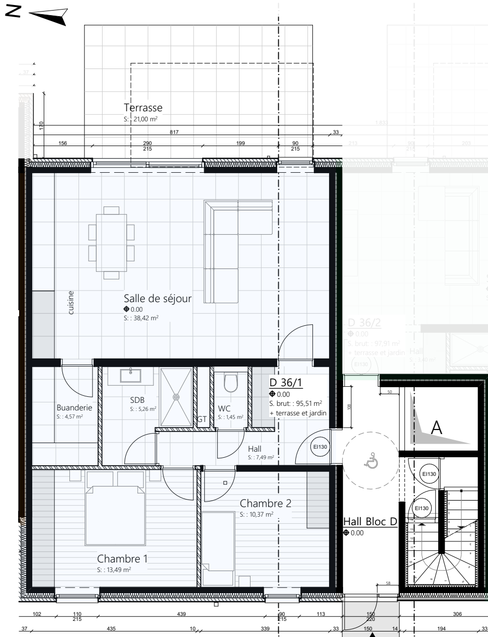
0. Rez-de-chaussée 1:100
