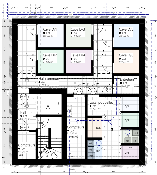
-1. Sous-sol 1:150
