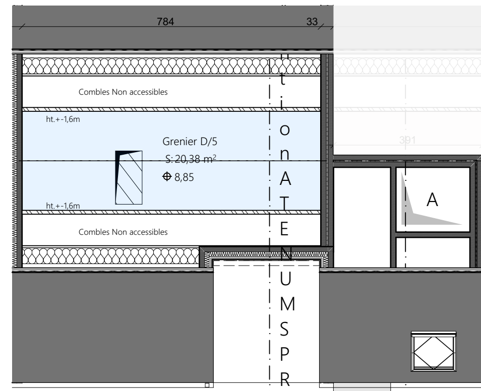
3. 3e Etage 1:100
