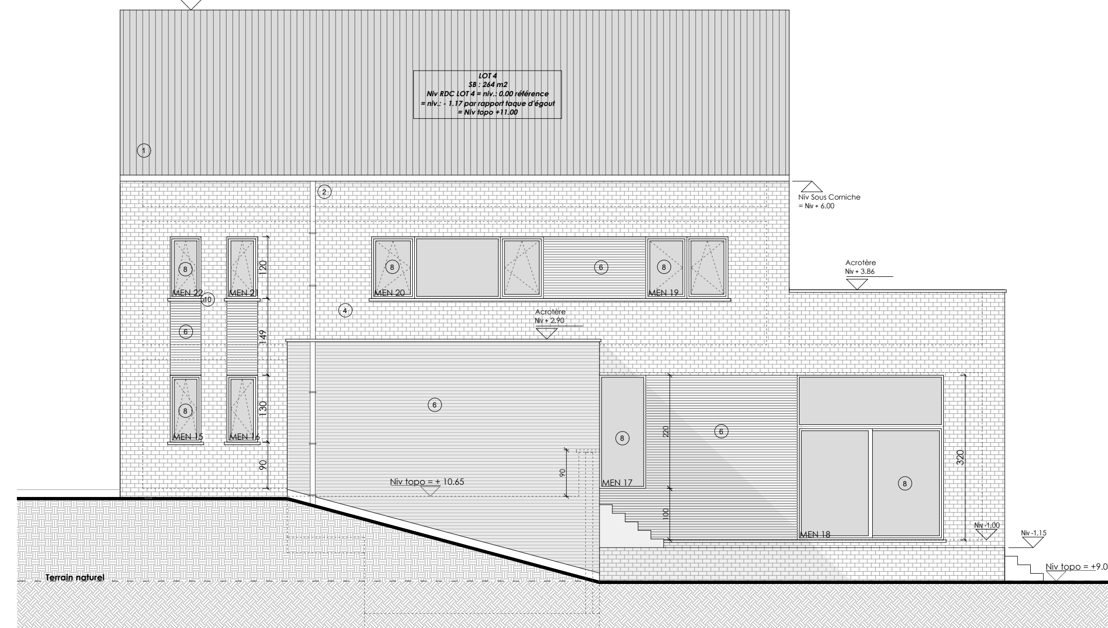
Facade latérale gauche 1/75
