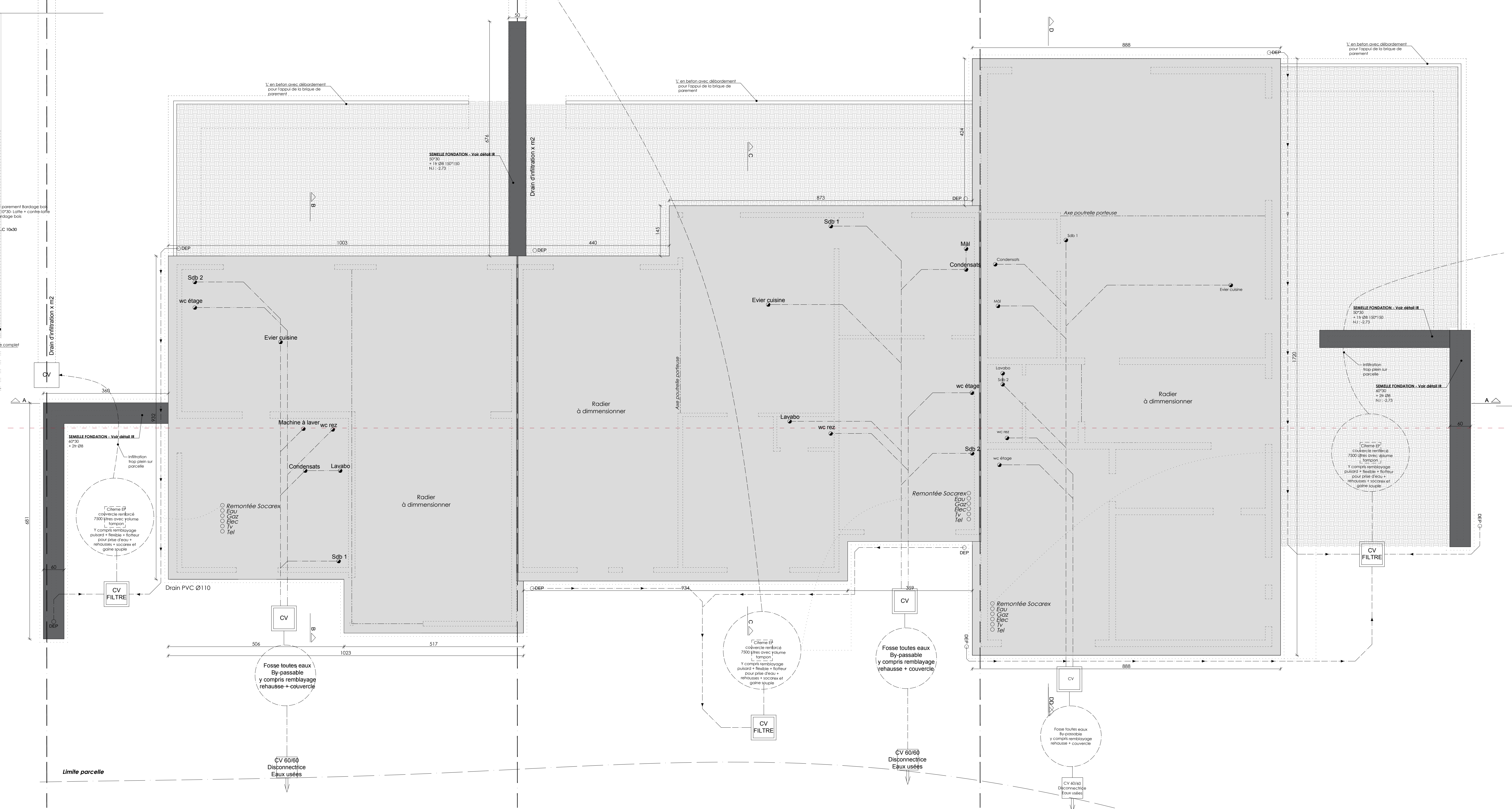
Façade latérale droite_ 1/75
