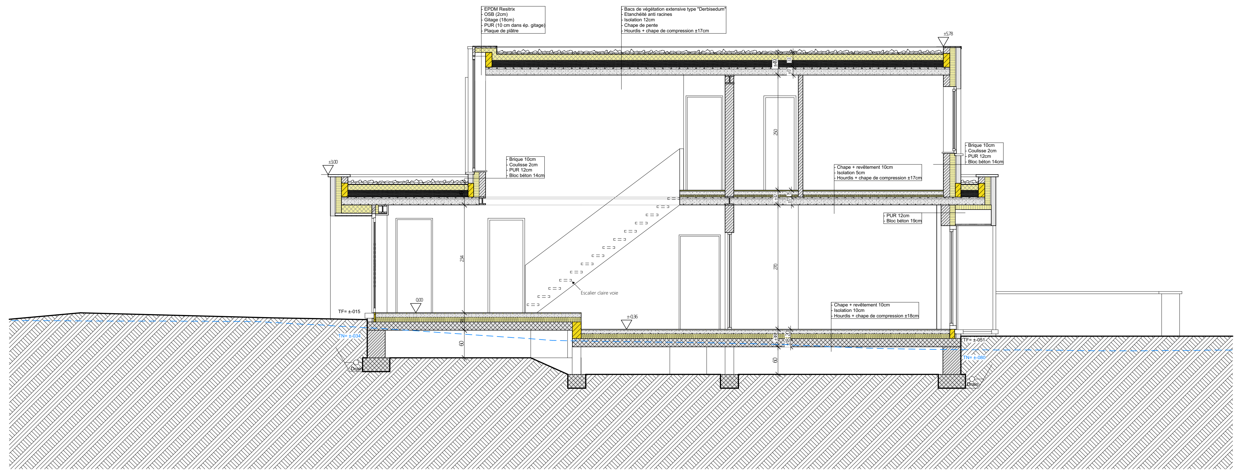
Coupe AA
