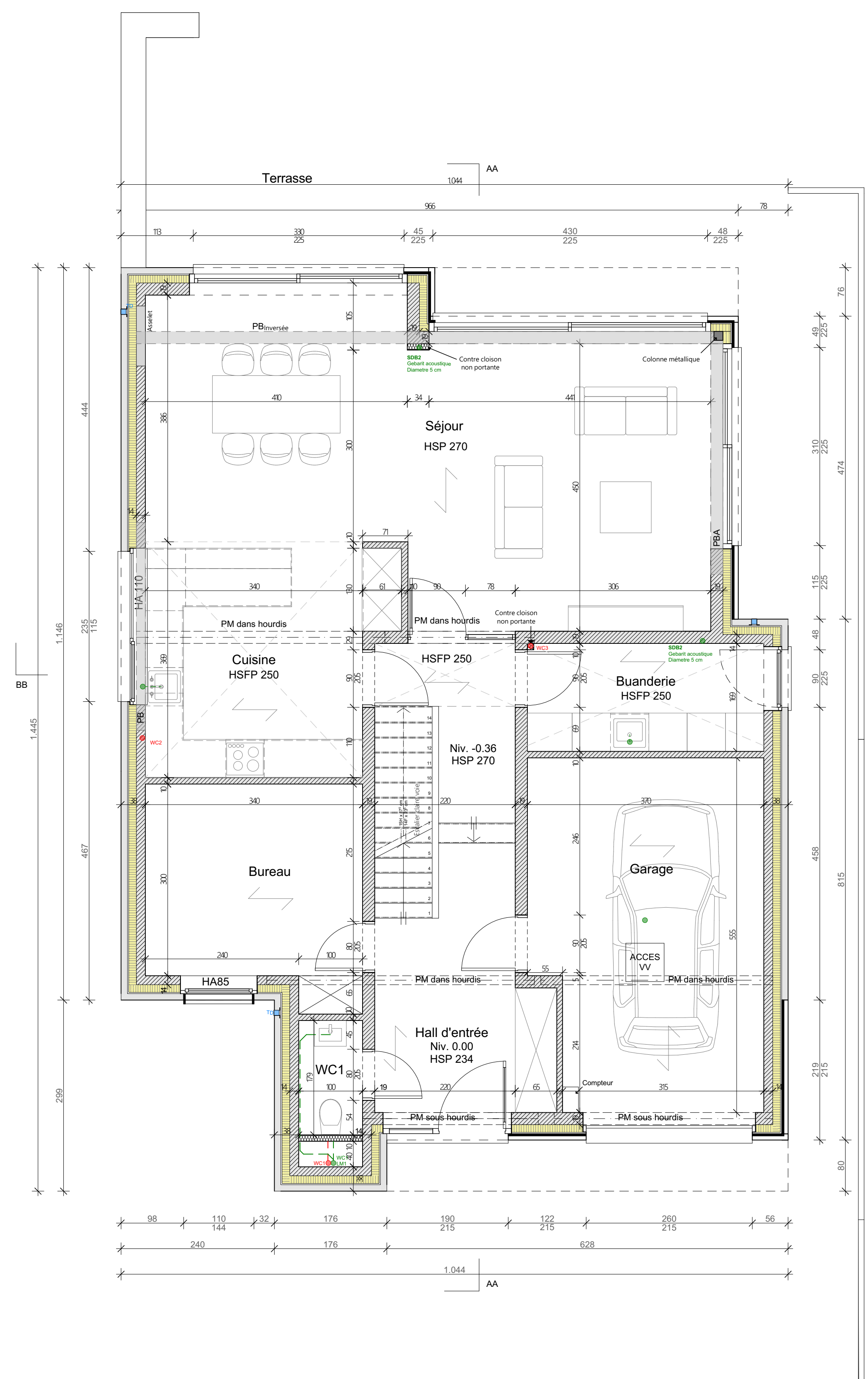
Rez-de-chaussée
