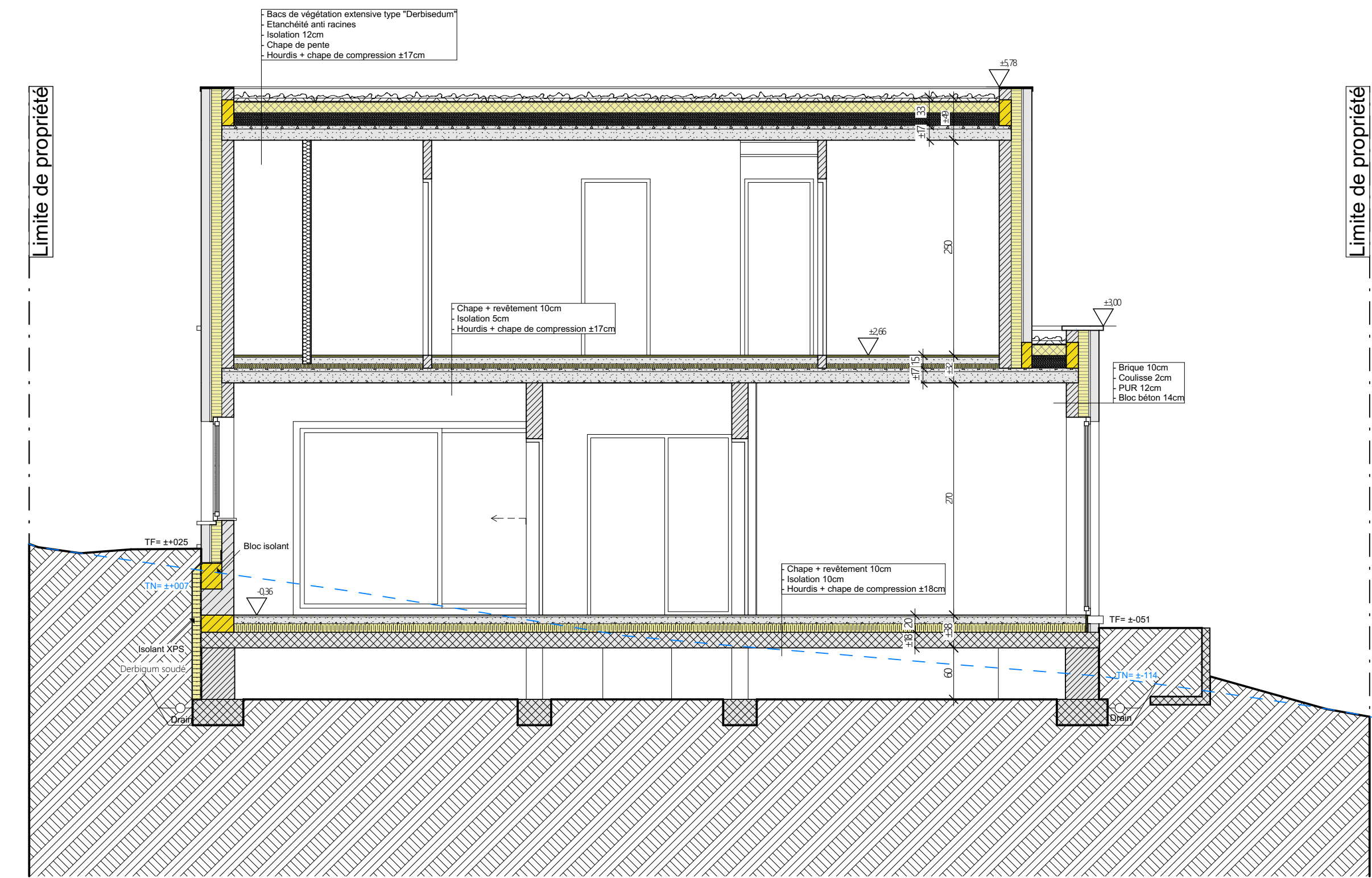
Coupe BB
