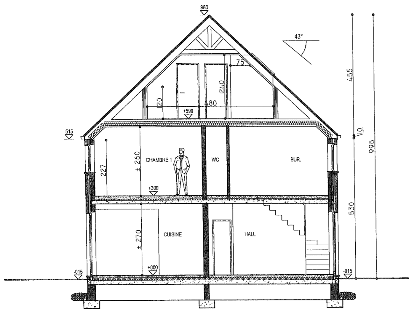
COUPE A - A
