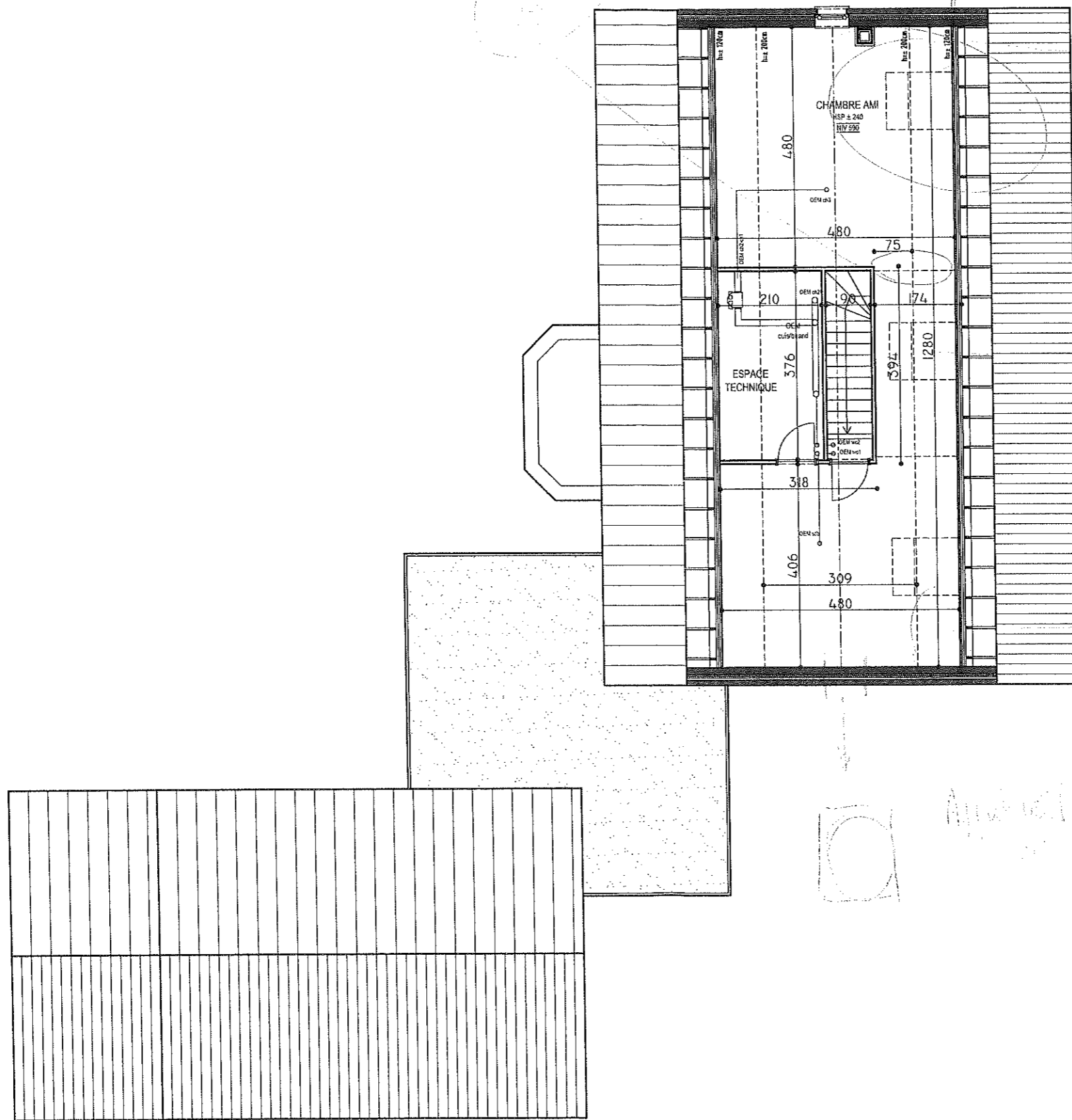
PLAN DU GRENIER
