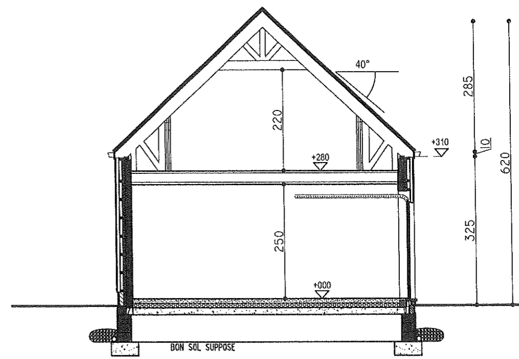
COUPE BB'
