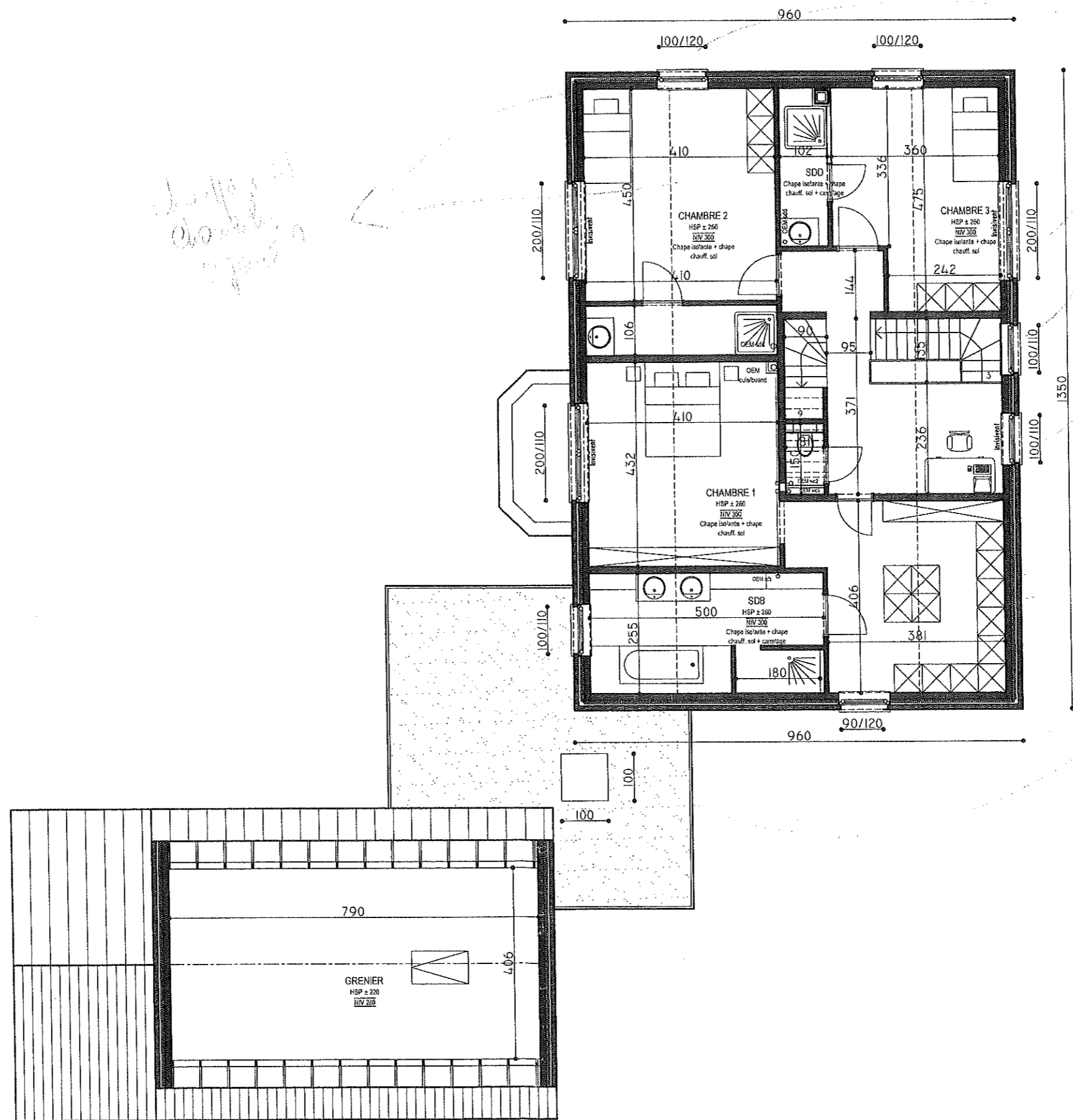
PLAN DE L'ETAGE
