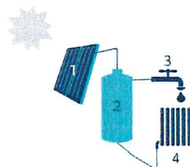
1. Zonnecollector | 2. Opslagvat zonneboiler | 3. Sanitair warm water | 4. Afgiftesysteem voor ruimteverwarming
