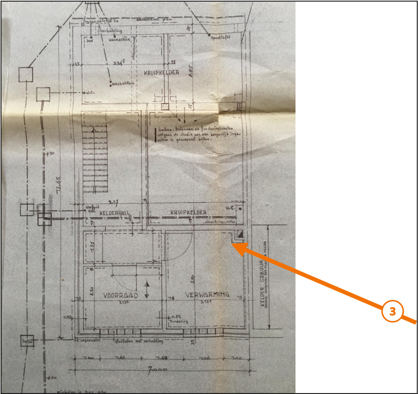
Legende van plan 1.3: Plan kelder
