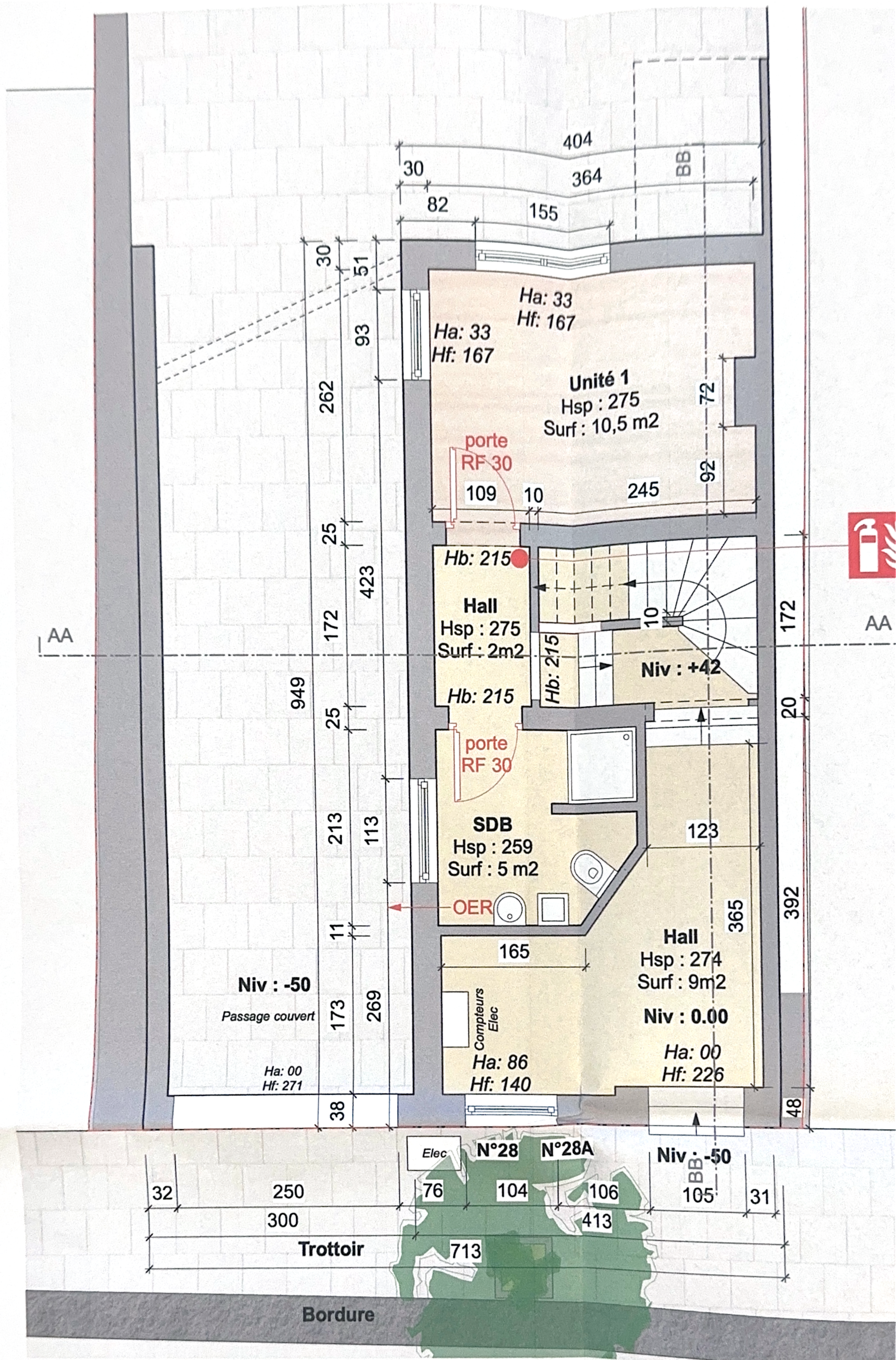
Plan Rez-de-Chaussée - Ech : 1/50
