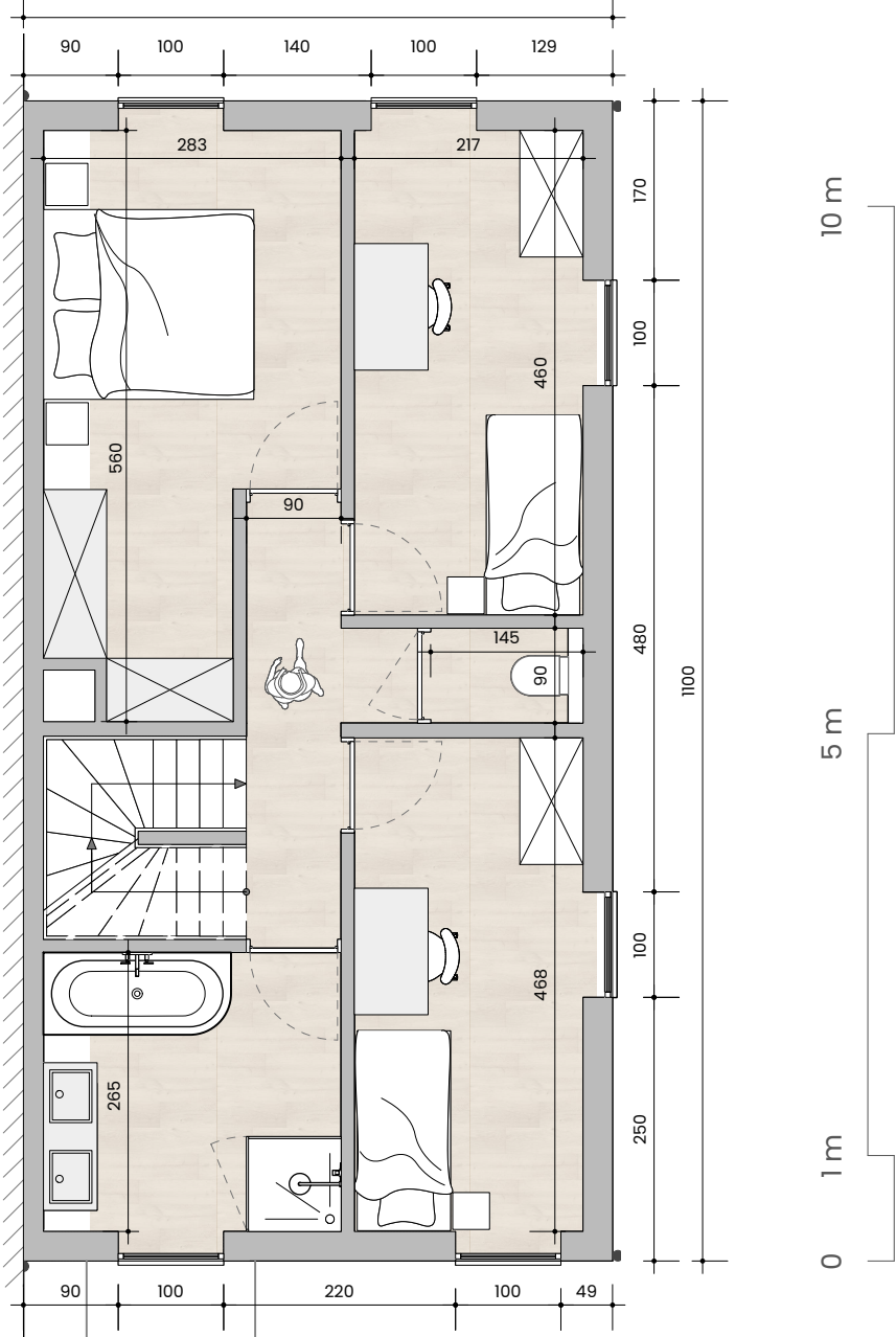
Verdiepingsplan +1
