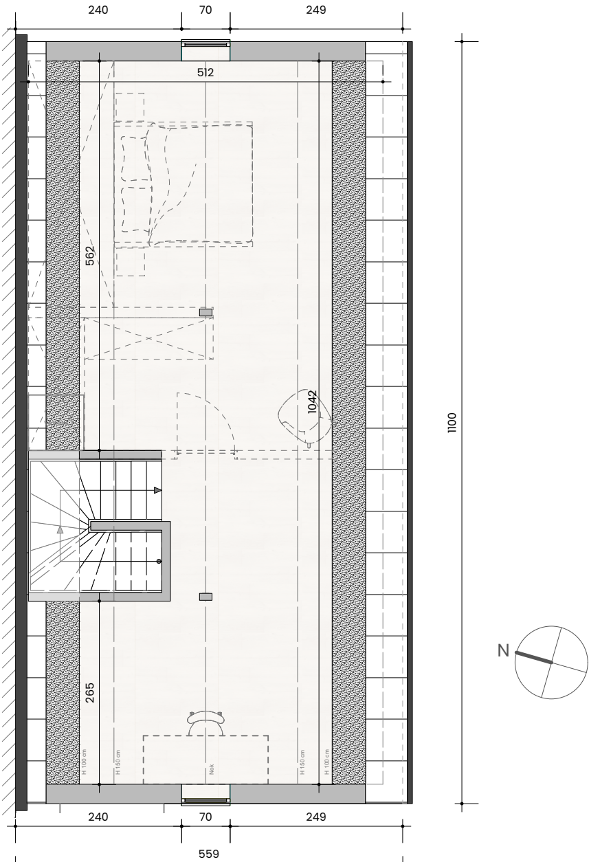
Verdiepingsplan +2 (casco)
