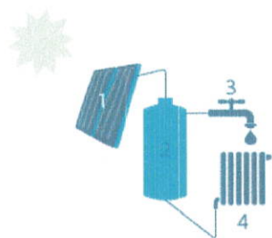
1. Zonnecollector | 2. Opslagvat zonneboiler | 3. Sanitair warm water | 4. Afgiftel element voor ruimteverwarming (optioneel)
