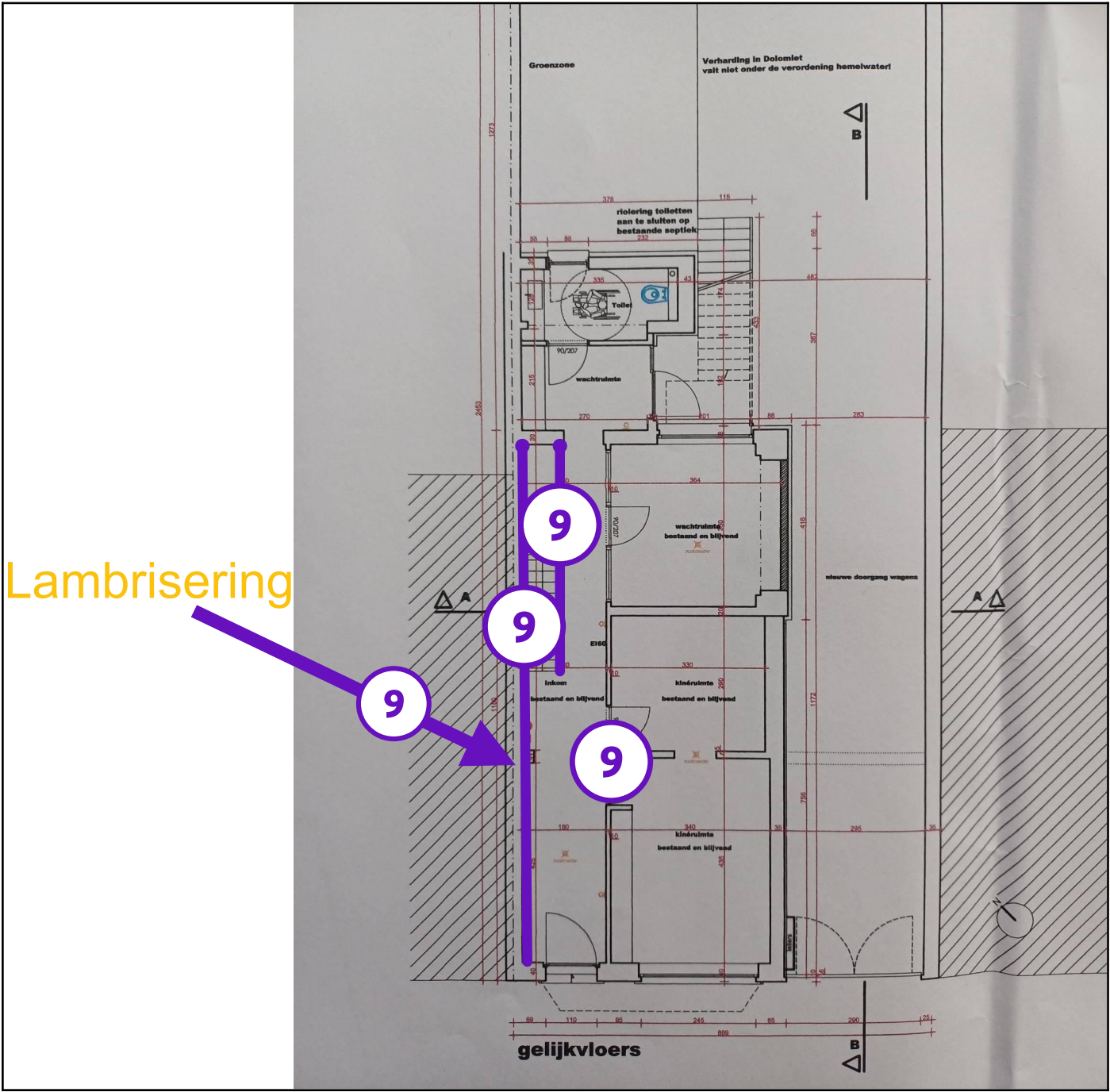
Legende van plan 1.4: Gelijkvloers - lambrisering
