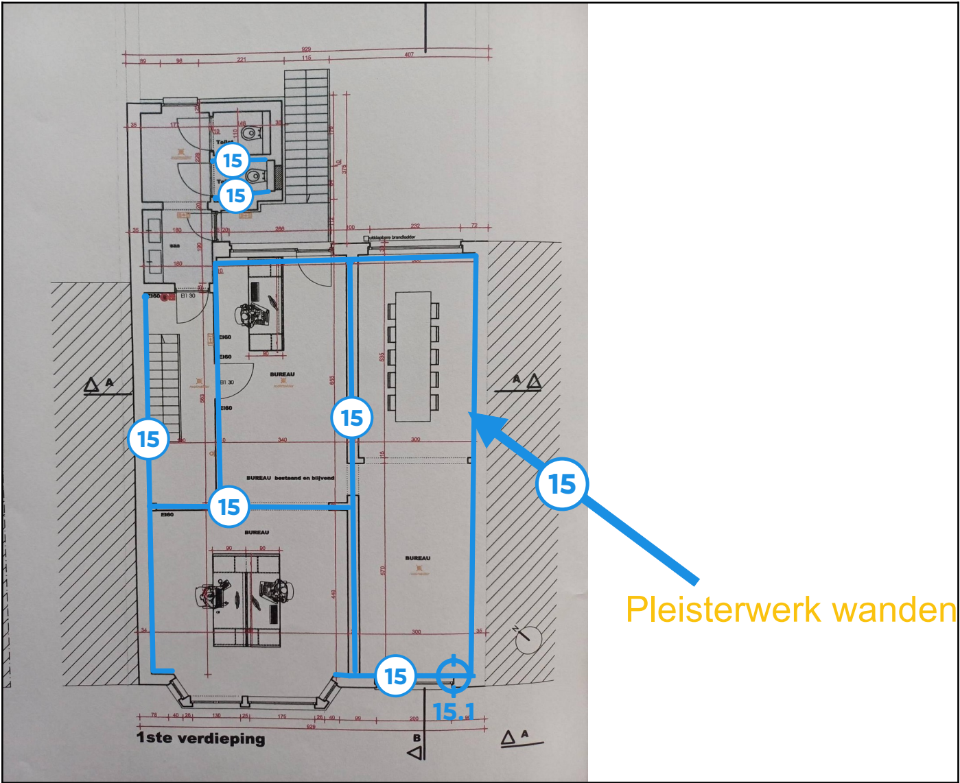
Legende van plan 1.10: 1ste verdieping - pleisterwerk wanden
