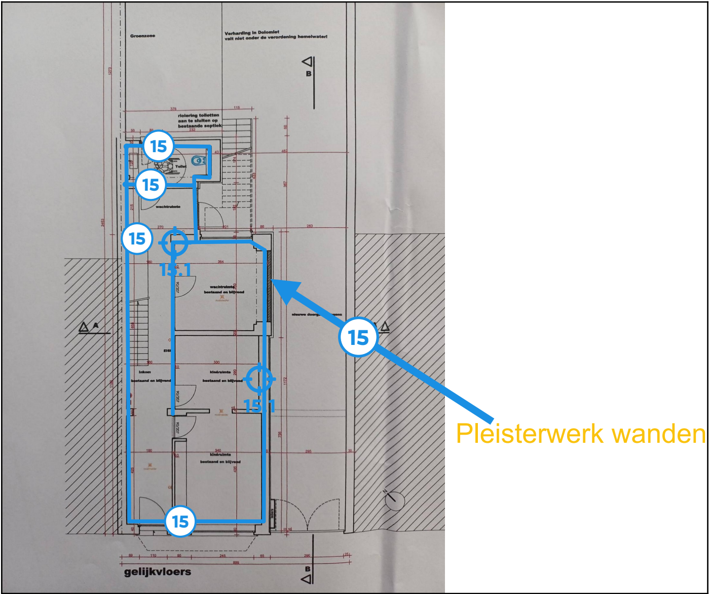
Legende van plan 1.6: Gelijkvloers - pleisterwerk wanden
