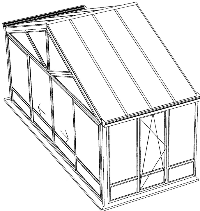
Vue Axono 2
