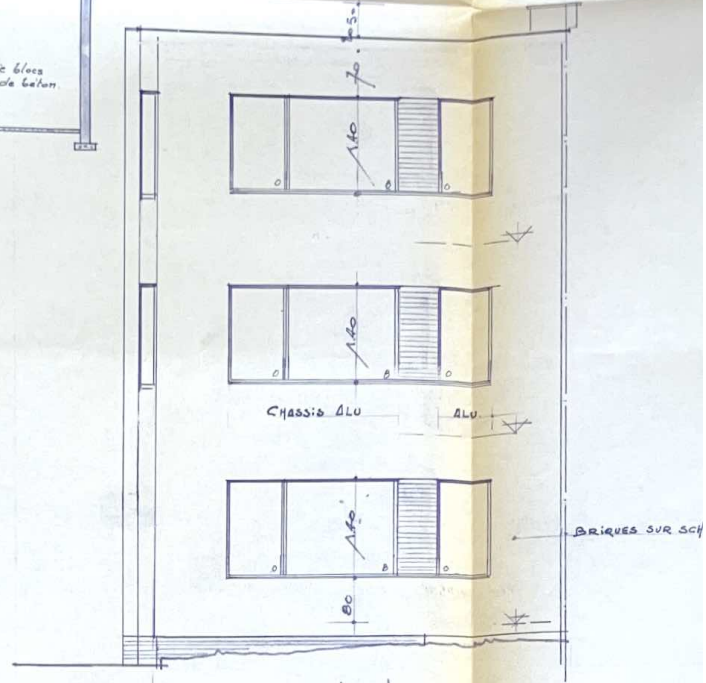
FACADE PRINCIPALE
