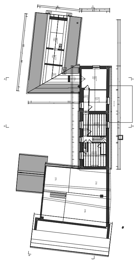
Etage 01
