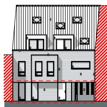
voorgevel
