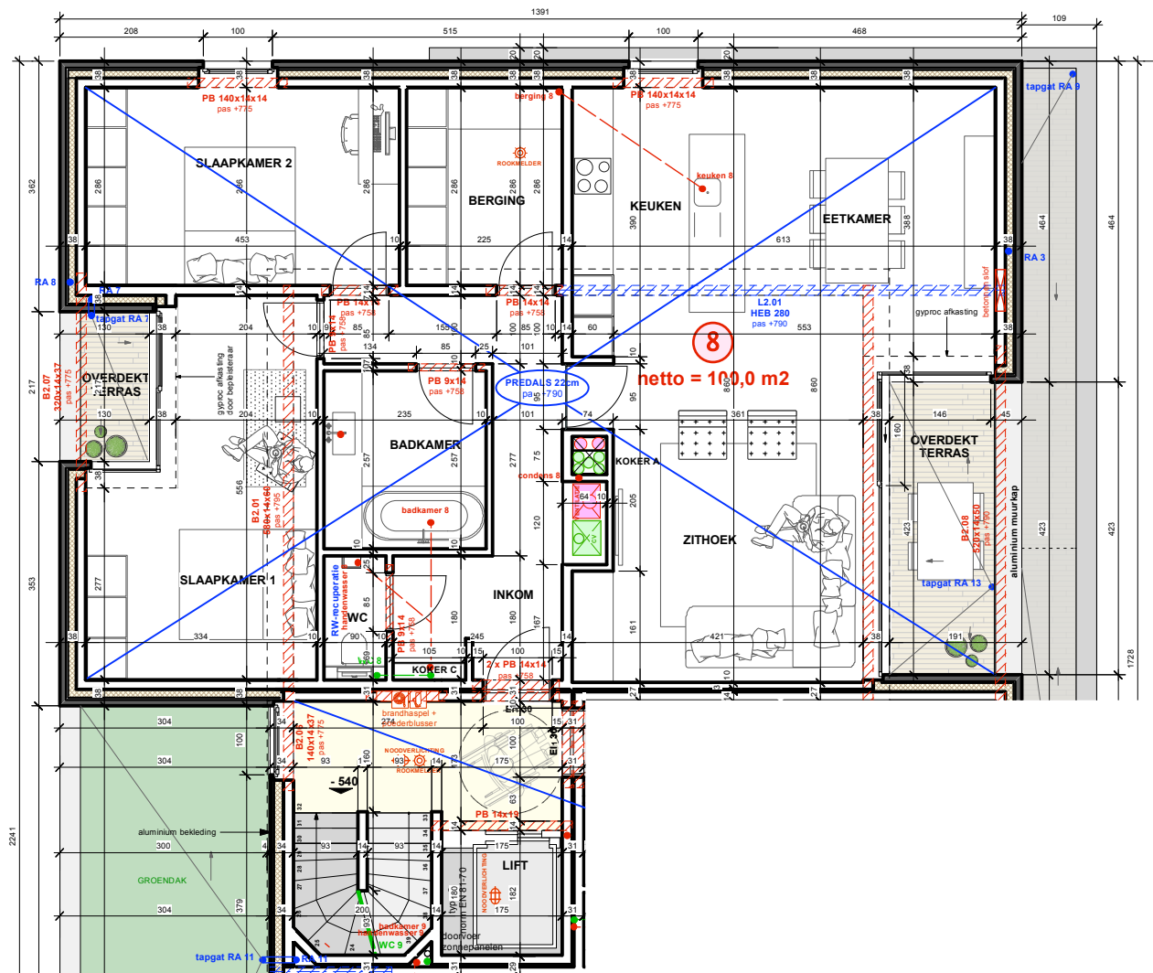
VERDIEPING +2 UNIT 2
