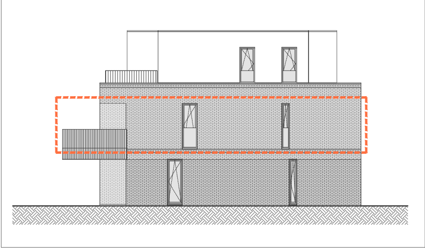
Zijgevel
