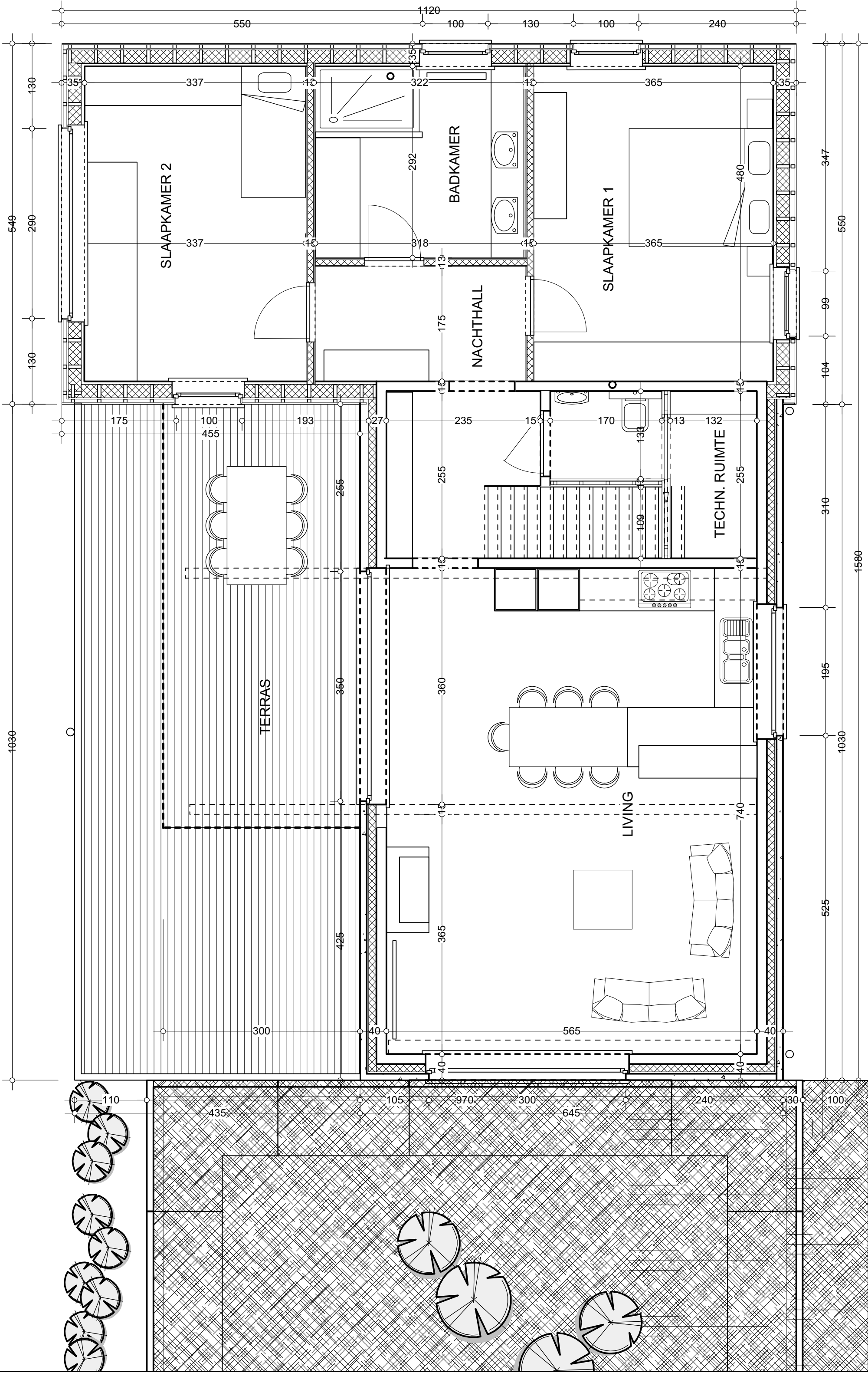
VERDIEPINGSPLAN nieuwe toestand
