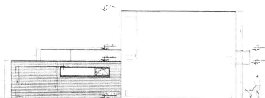
ELEVATION LATÉRALE GAUCHE - 1/50ème
