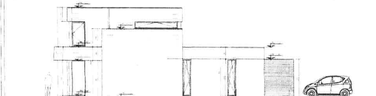
ELEVATION LATÉRALE DROITE - 1/50ème
