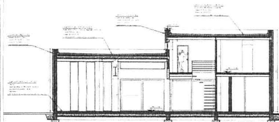
COUPE BB - 1/50ème
