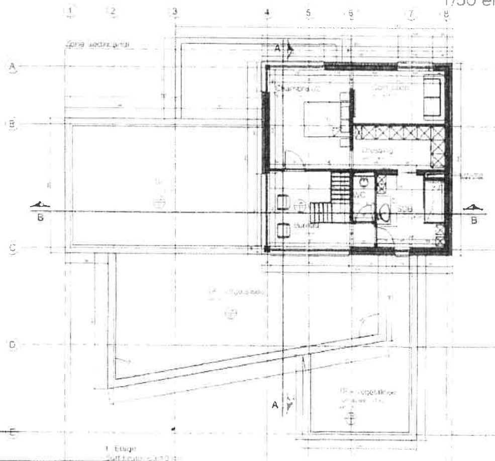
PLAN 1° ETAGE 1/50 ème
