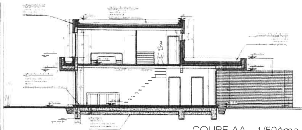
COUPE AA - 1/50ème
