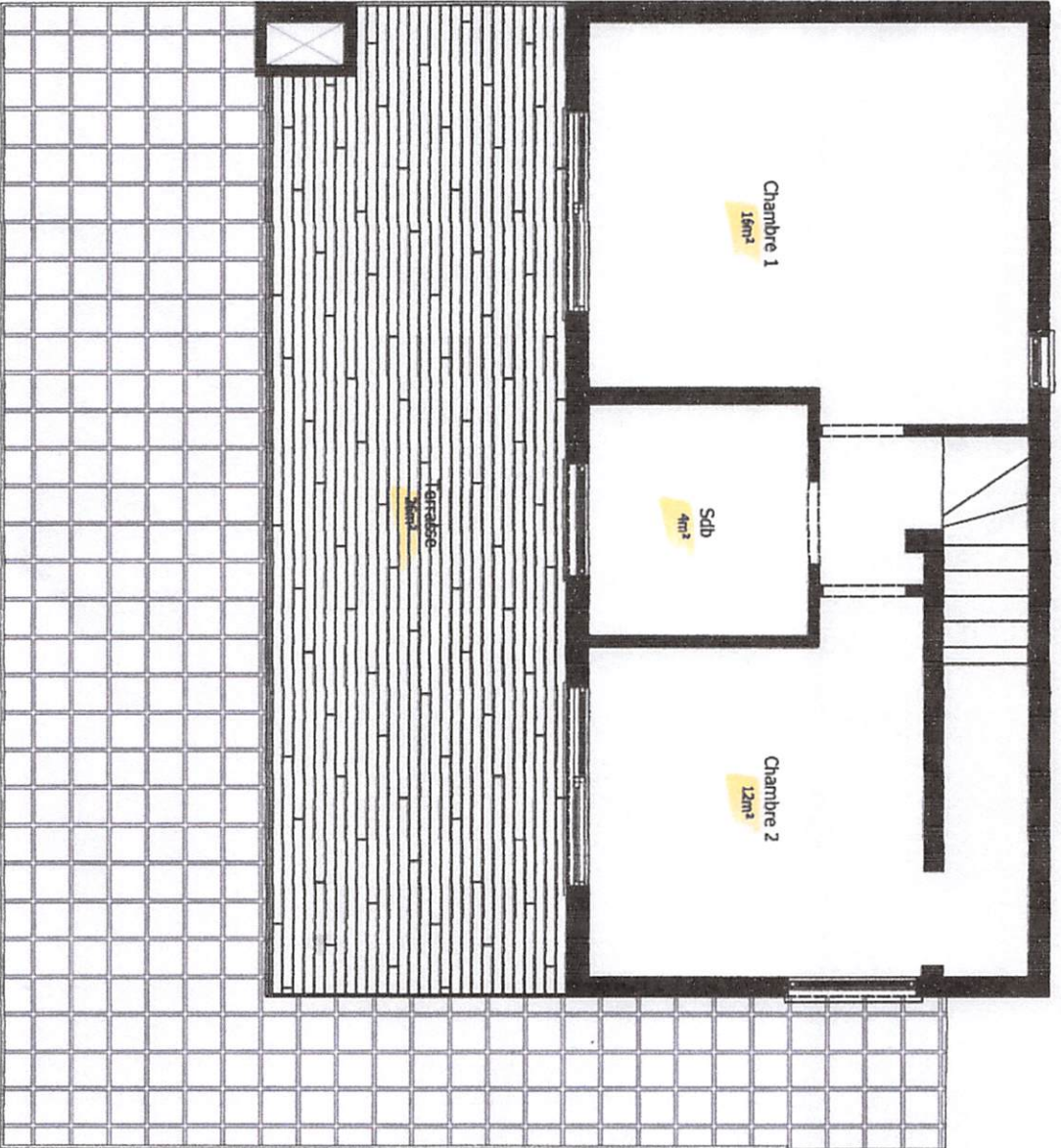
Plan Etage 2 Echelle 1/50
