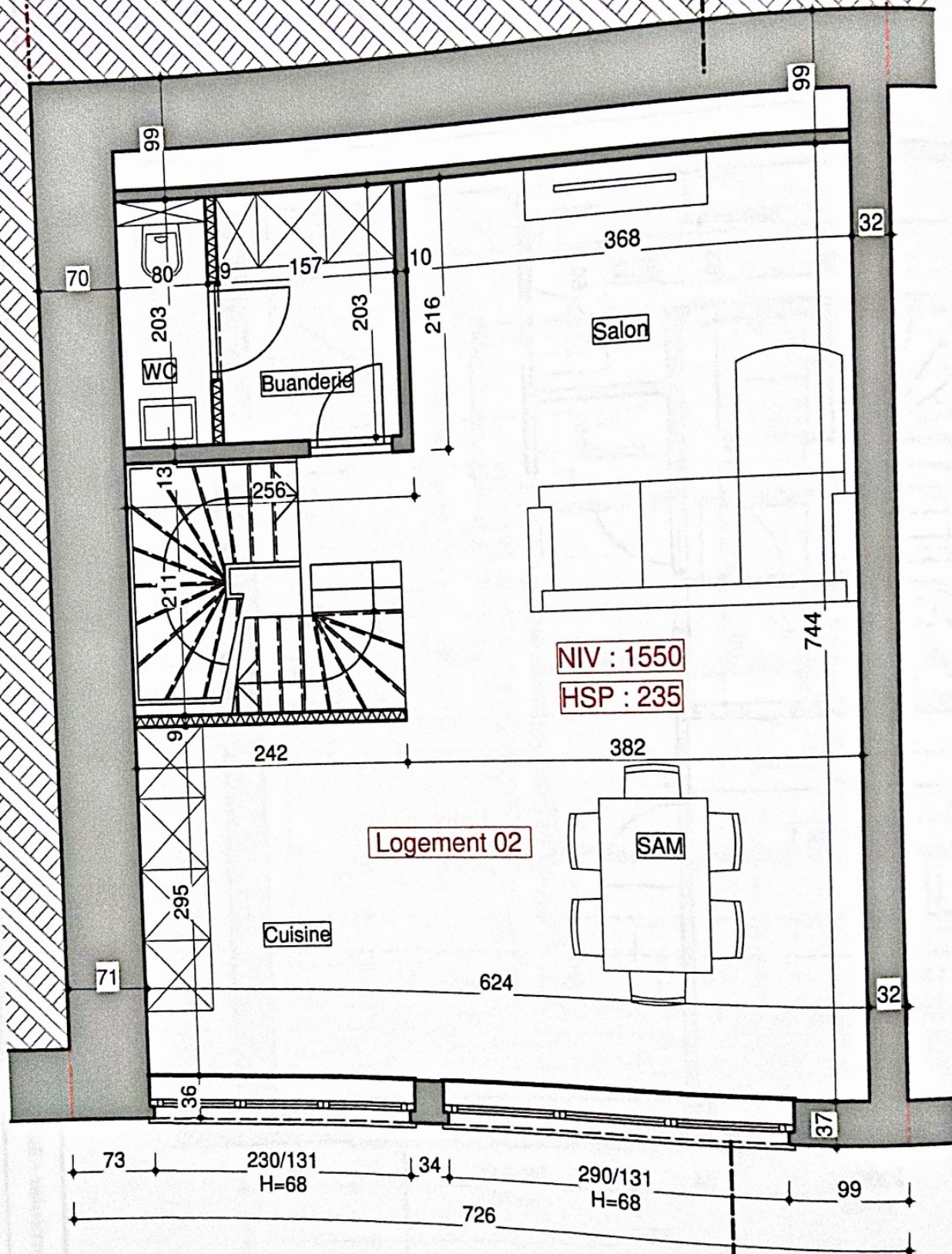
Plan projeté: Etage 02
