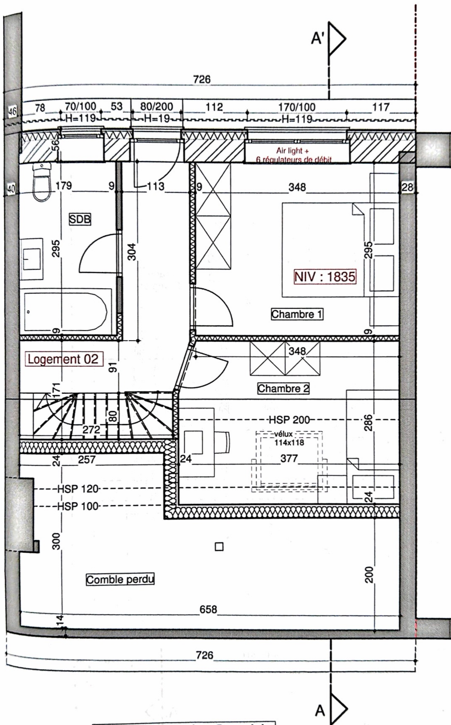
Plan projeté : Comble
