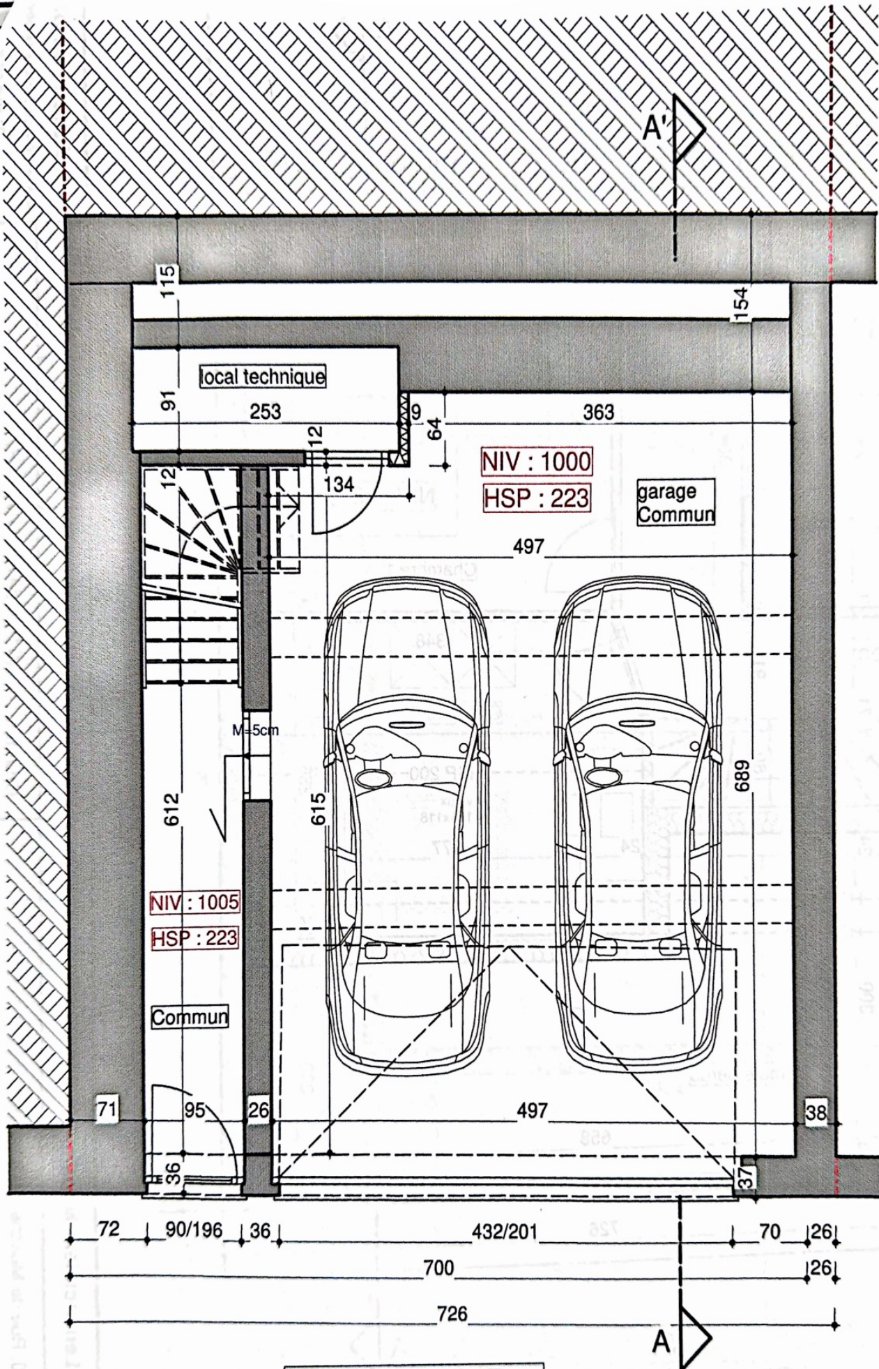
Plan projeté: Rez
