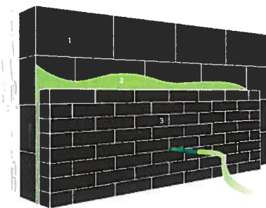
1. Dragende muur | 2. Ingeblazen isolatie | 3. Gevelsteen / gevelbekleding
