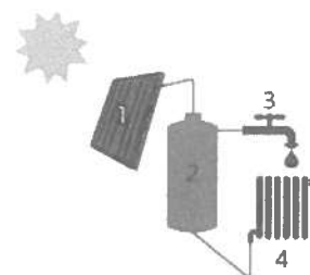
1 Zonnecollector | 2 Opslagvat zonneboiler | 3 Sanitair warm water | 4 Afgiftedelement voor ruimteverwarming (radiator)
