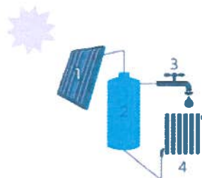
1 Zonnecollector (2) Opslagvat voor warm water (3) Zonnepomp (4) Radiator
