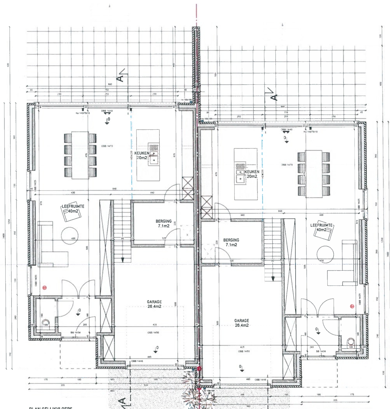
PLAN GELIJKVLOERS bruto opp. 120 m 2
