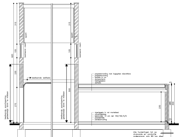
DOORSNEDE A-B
