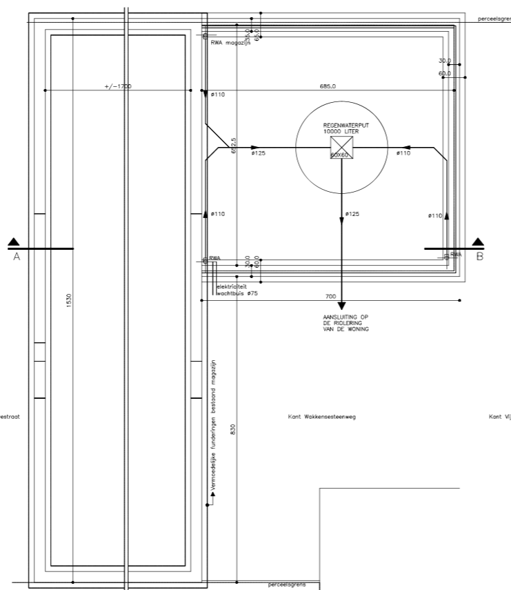
FUNDERING EN RIOLERING
