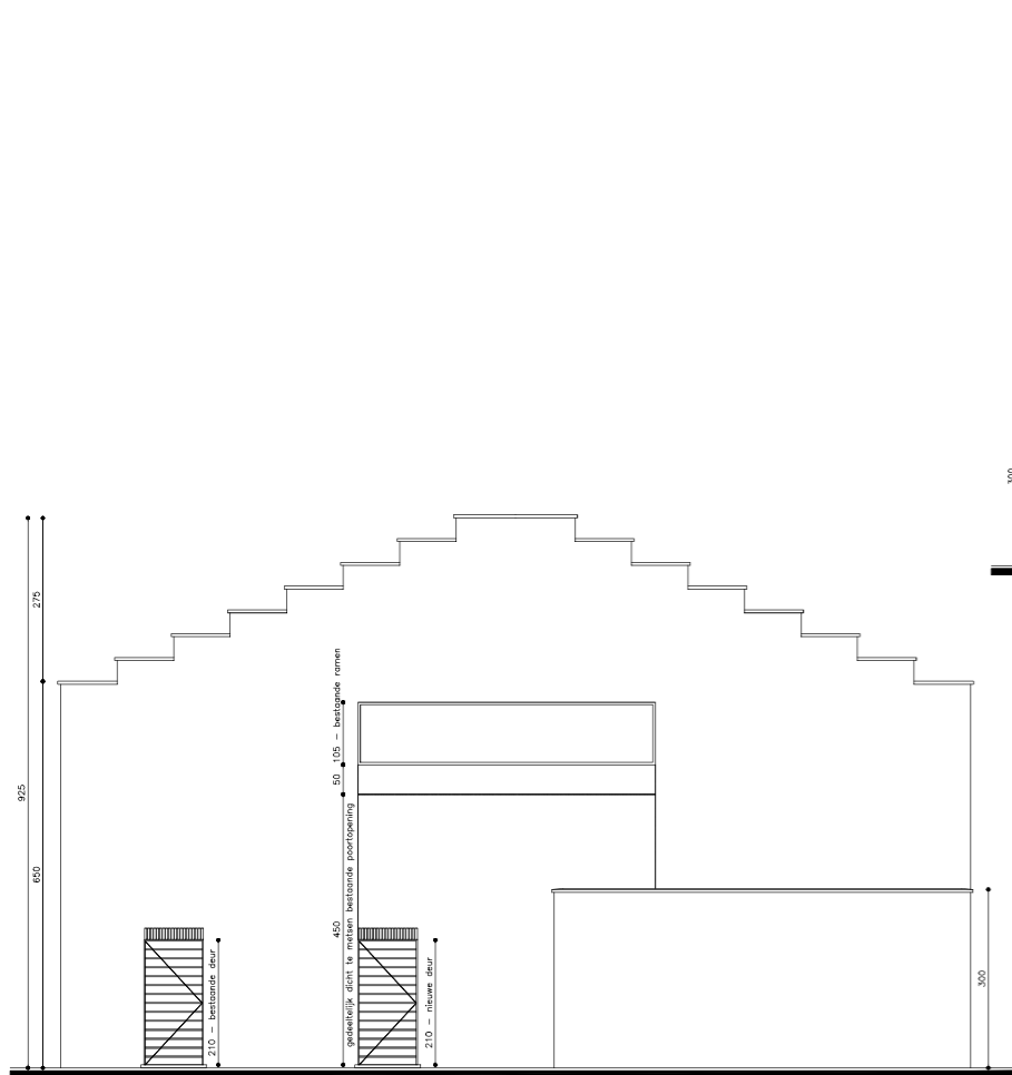
NOORDWESTGEVEL
