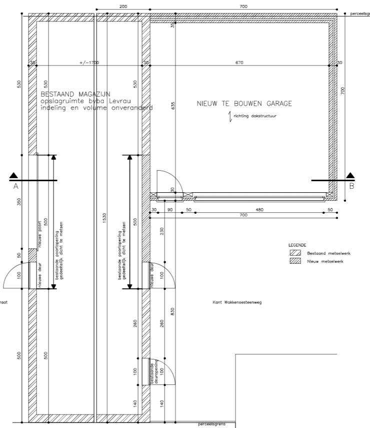
GRONDPLAN
