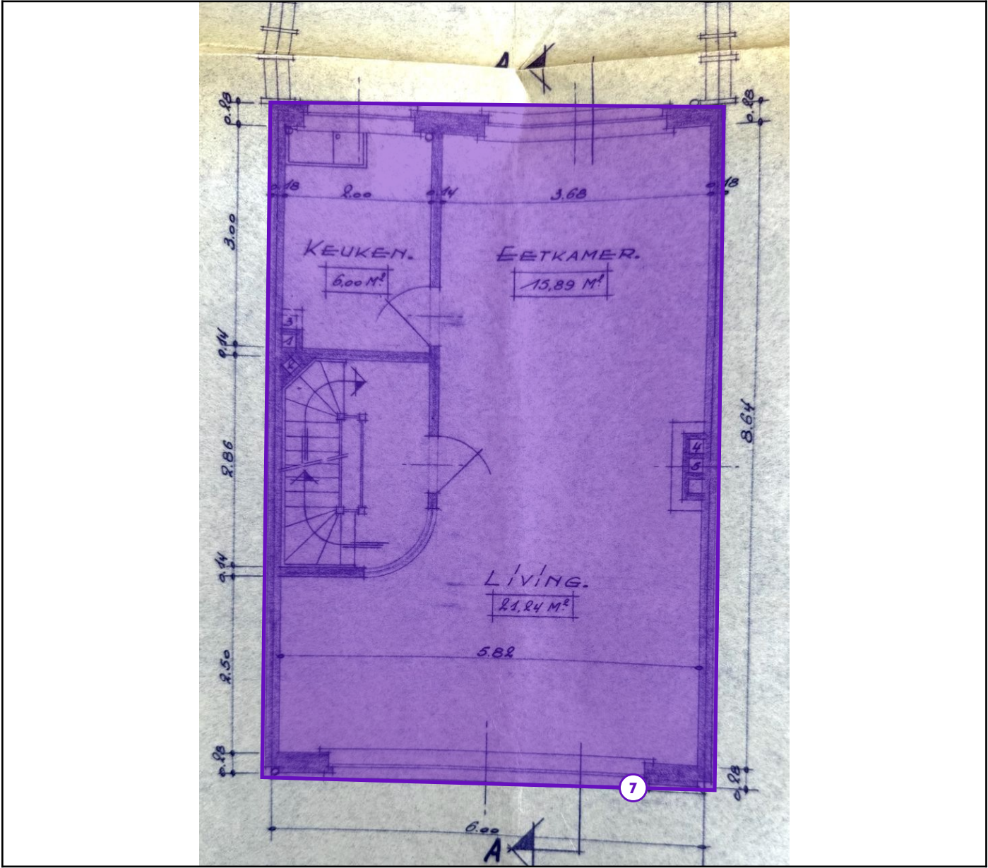
Legende van plan 1.4: Verdiep 1
