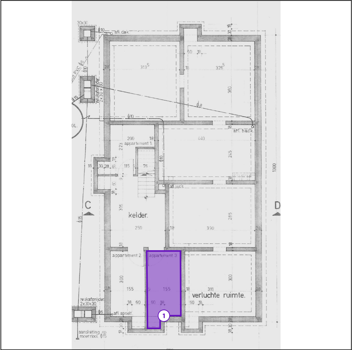
Legende van plan 1.3: Kelderverdieping
