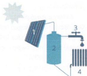
1. Zonnecollector | 2. Opslagvat, zonneboiler | 3. Sanitair warm water | 4. Afsluit-element voor ruimteverwarming, optioneel
