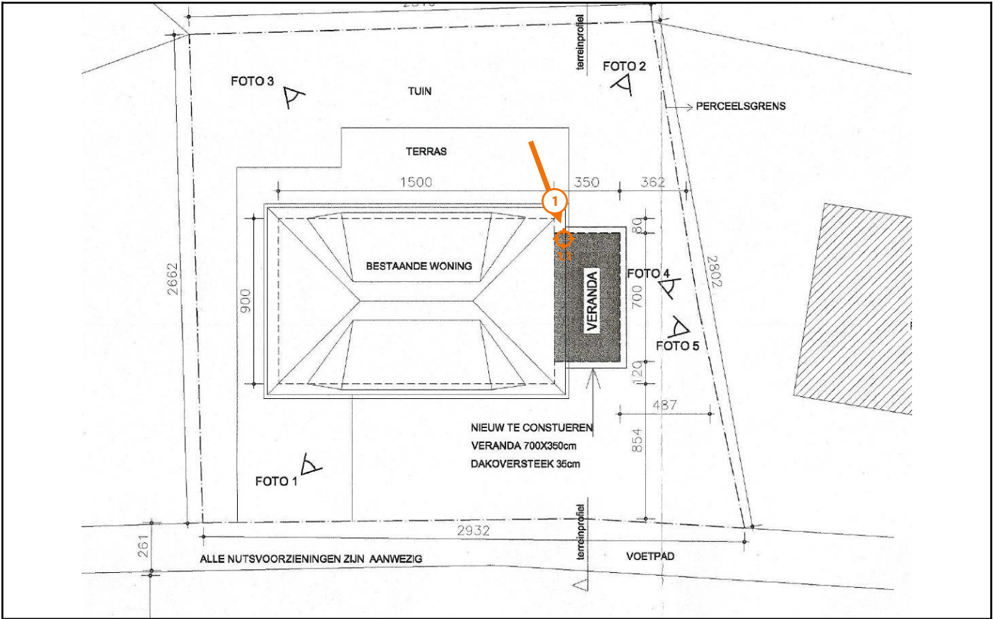
Legende van plan 1.1: dakplan Mezenlaan 12 WILRIJK
