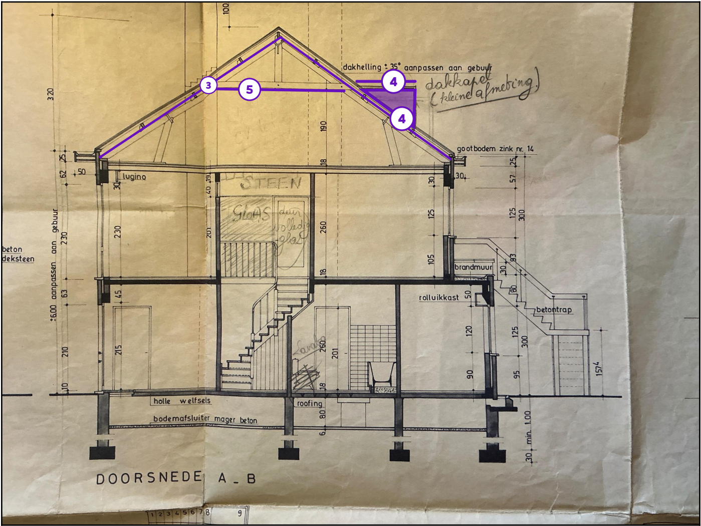
Legende van plan 1.6: Doorsnede
