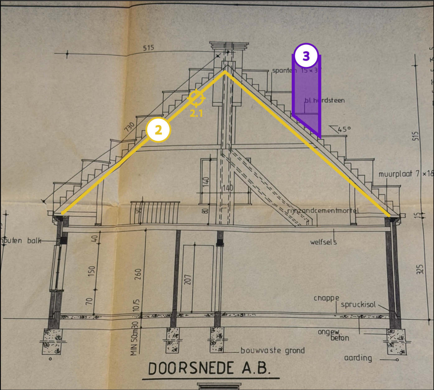
Legende van plan 1.3: Doorsnede huis
