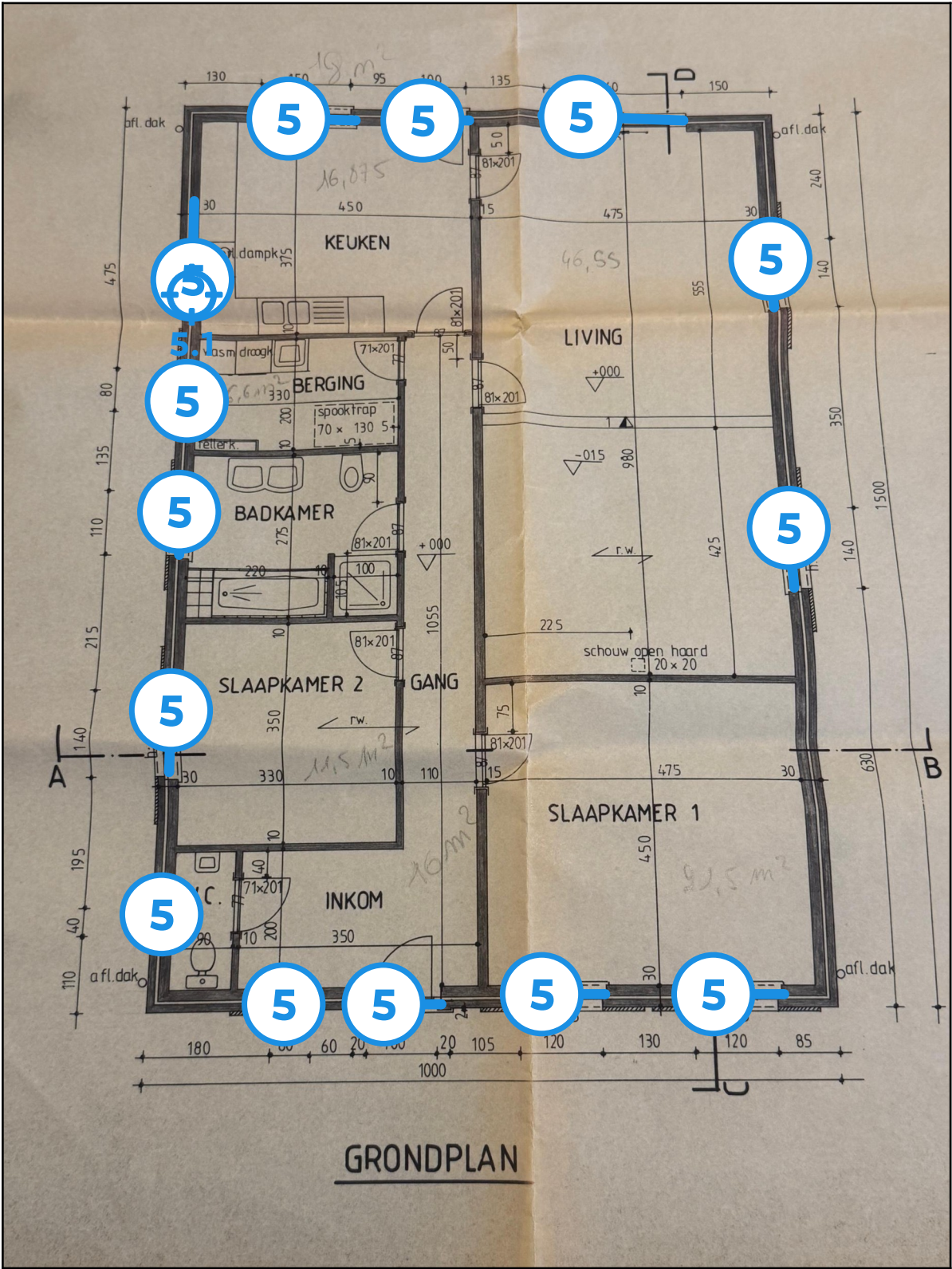
Legende van plan 1.6: Gvl - Mastiek ramen
