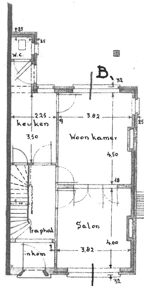
GELIJKVLOERS
