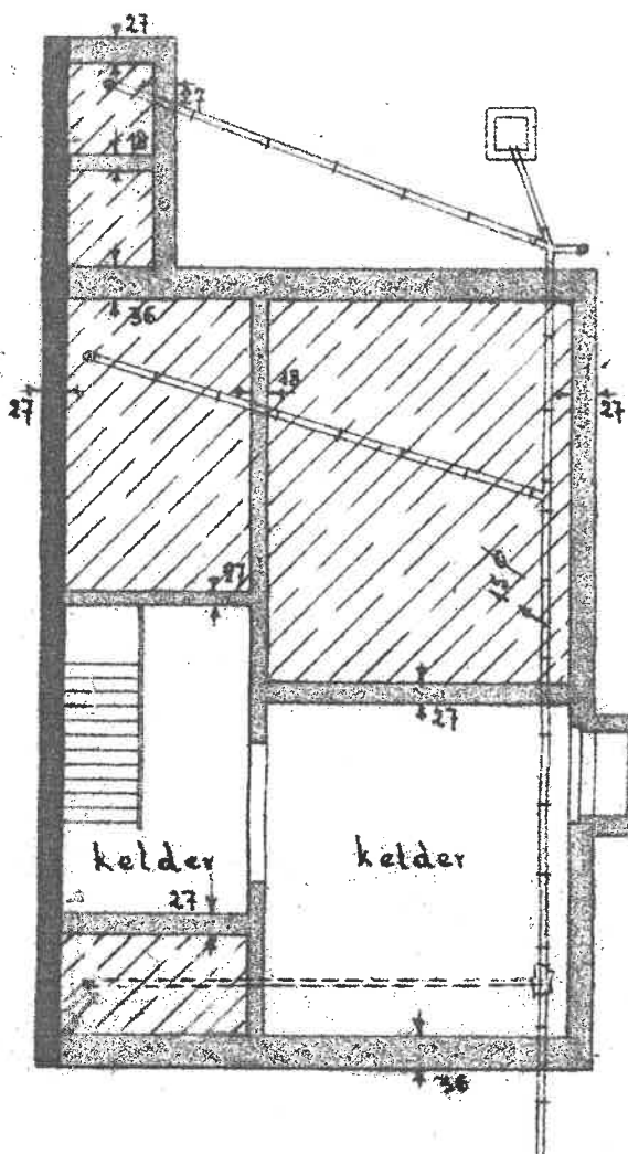
GRONDPLAN
