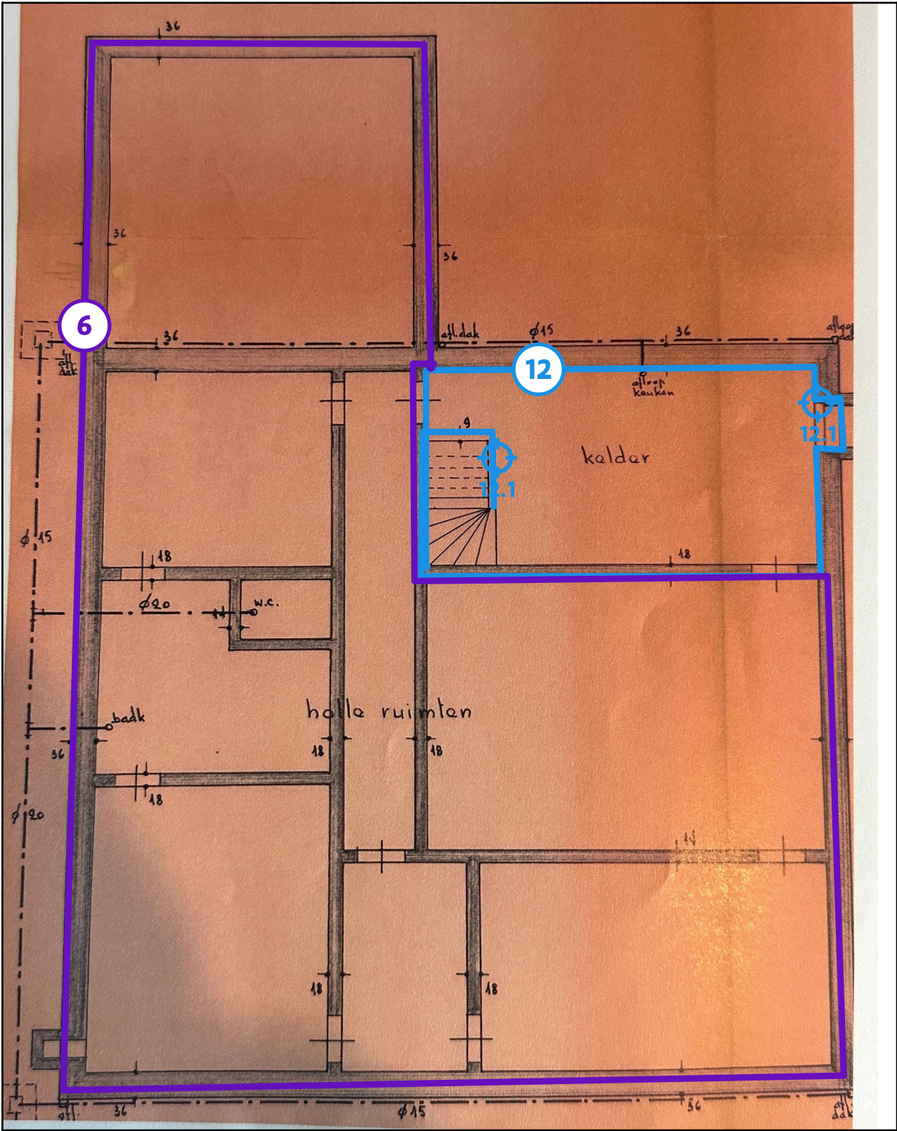
Legende van plan 1.1: Kelder-kruipkelder plan
