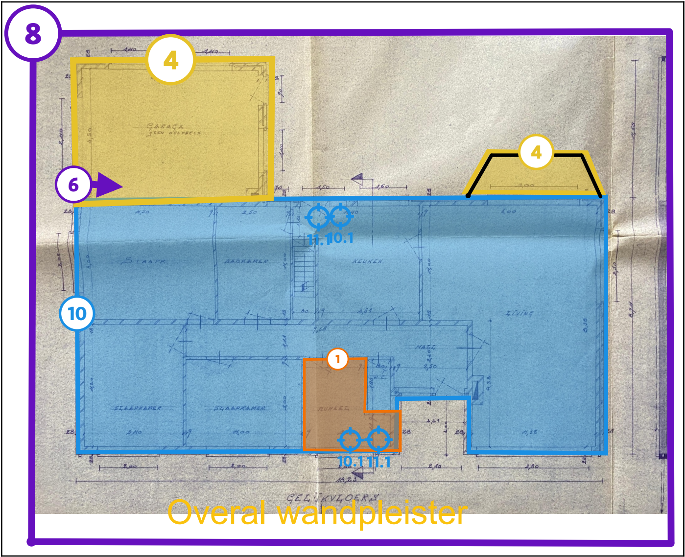
Legende van plan 1.2: Gelijkvloers plan
