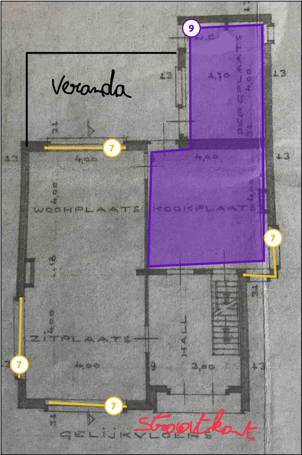
Legende van plan 1.7: Gelijkvloers
