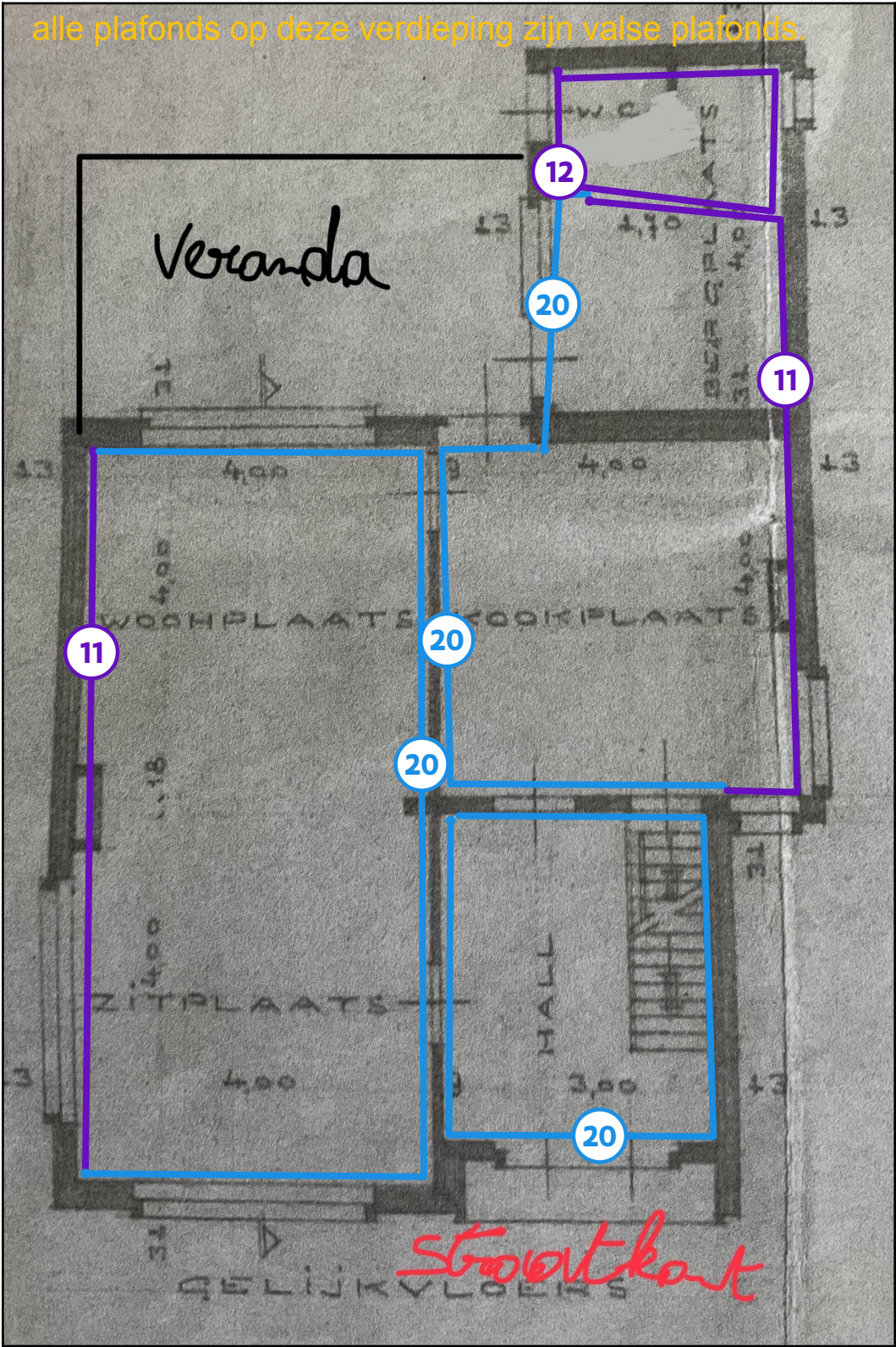
Legende van plan 1.5: Gelijkvloers
