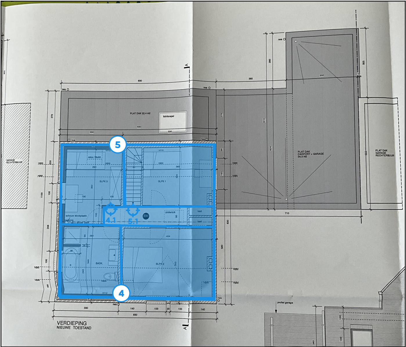
Legende van plan 1.6: verdieping pleisterwerk
