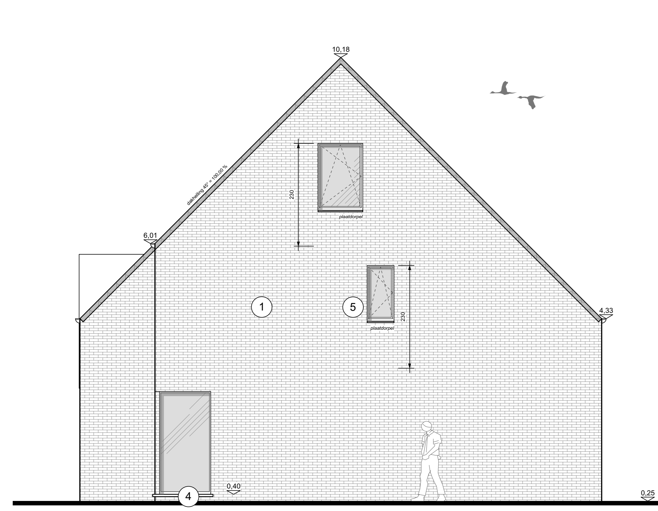
Lot 7 - zijgevel rechts
