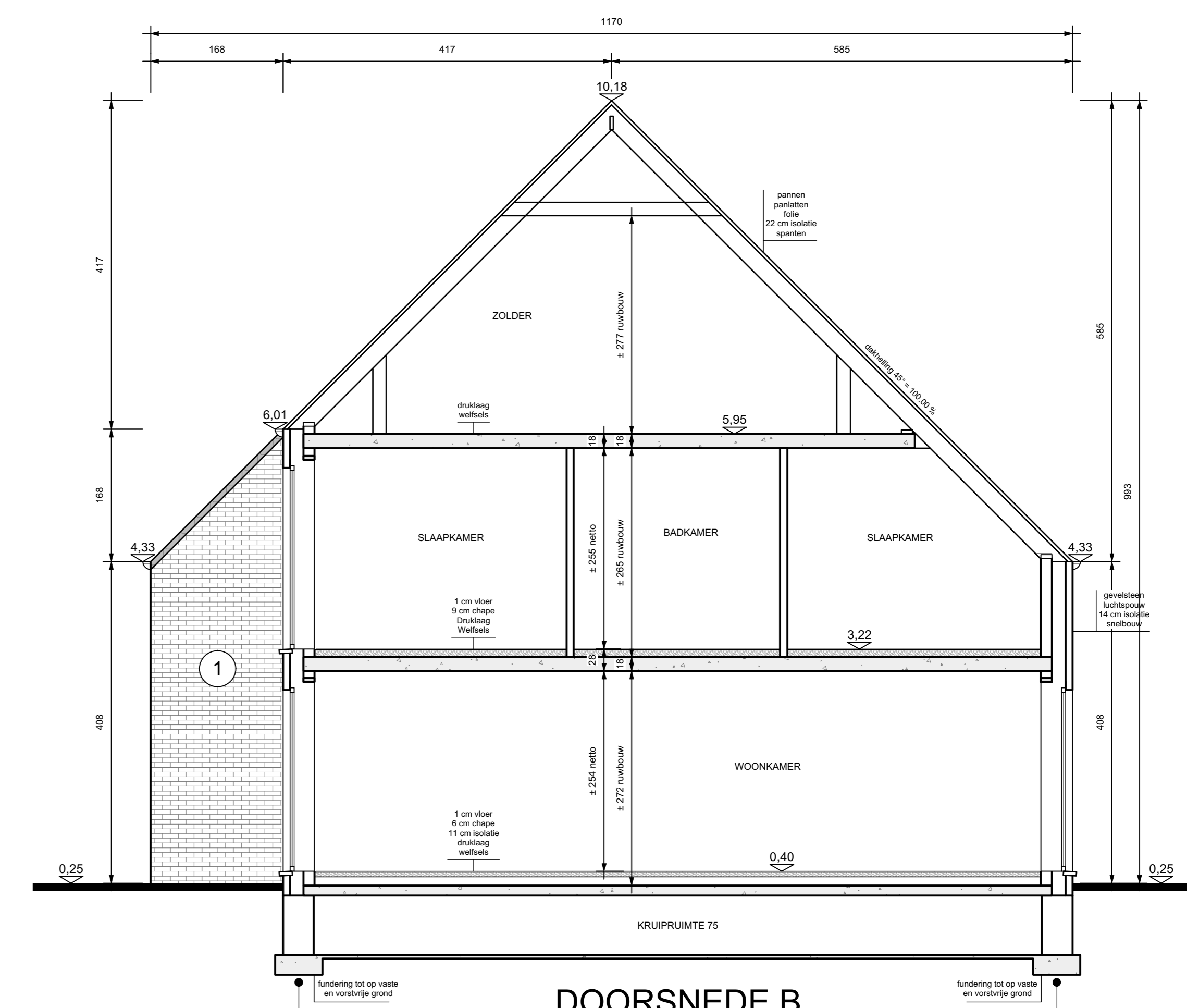
DOORSNEDE B
