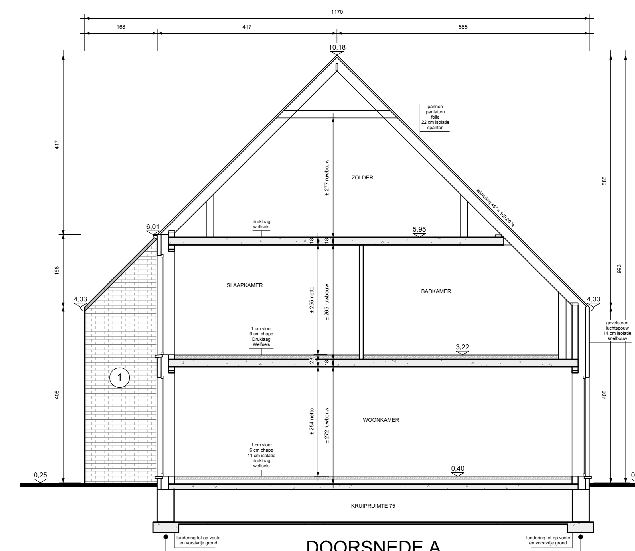
DOORSNEDE A
