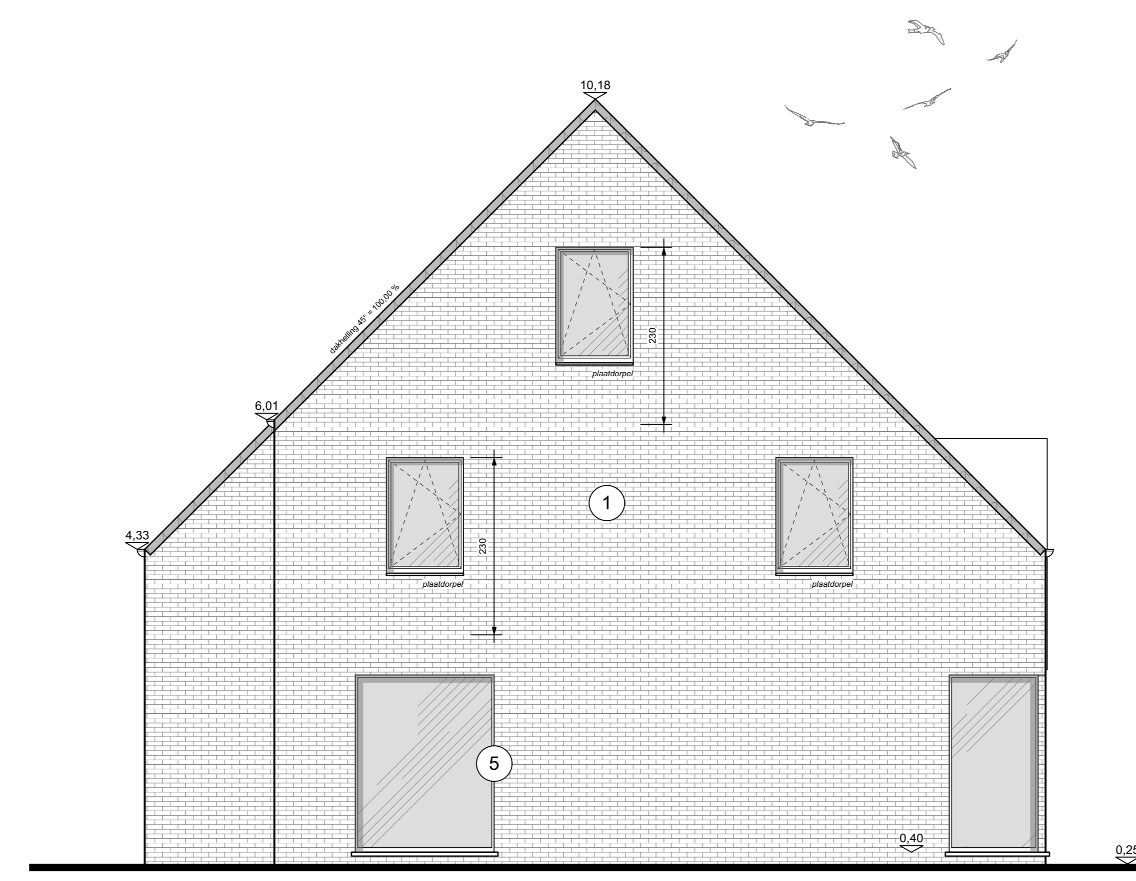
Lot 1 - zijgevel links
