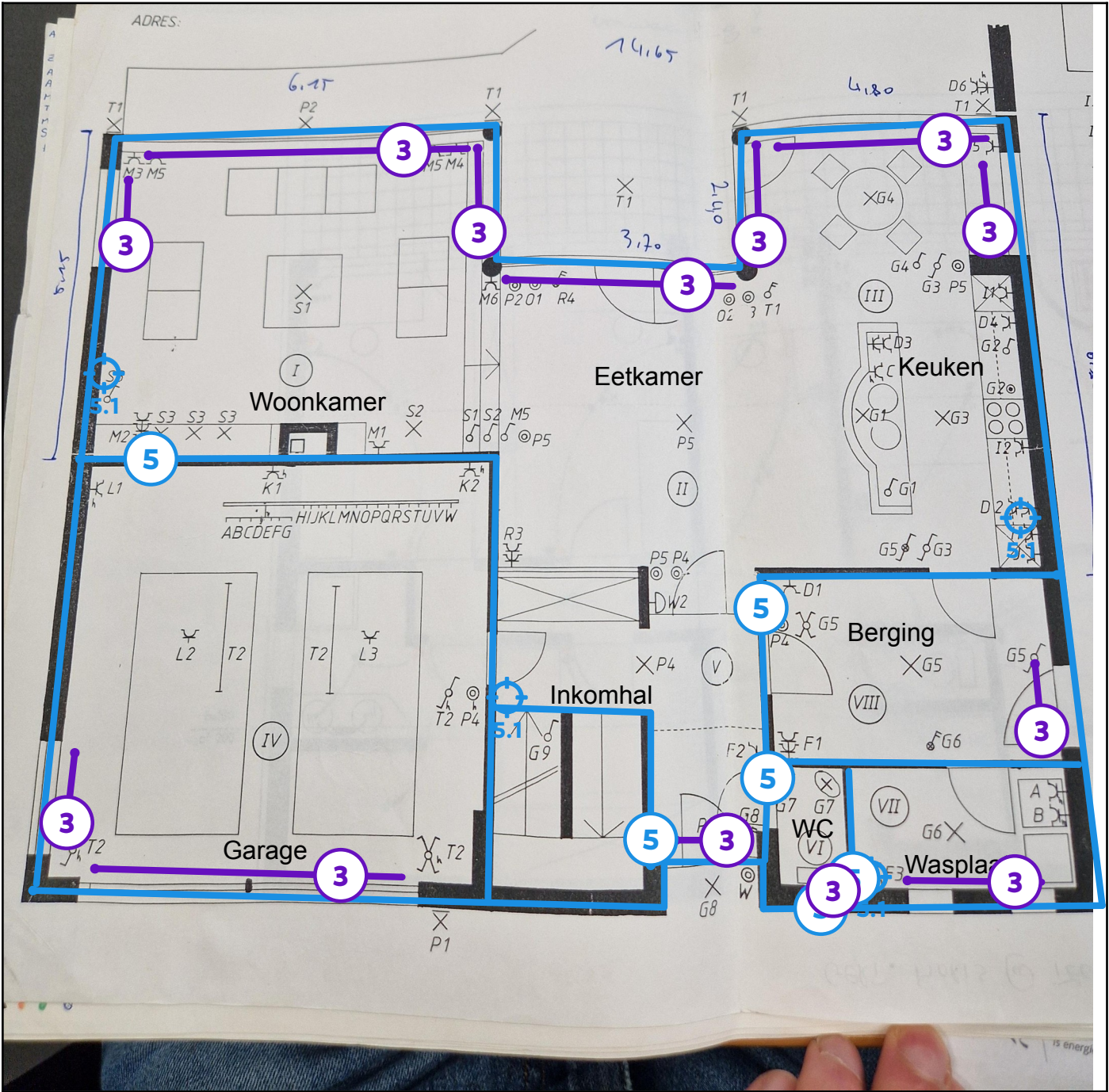
Legende van plan 1.1: Plan gelijkvloers
