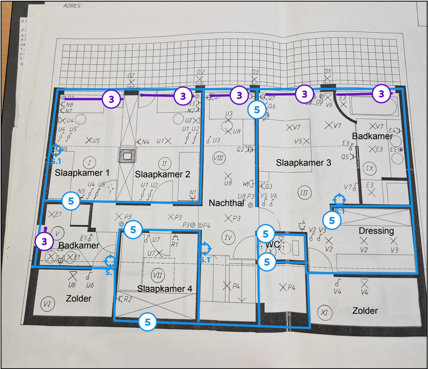
Legende van plan 1.3: Plan verdieping
