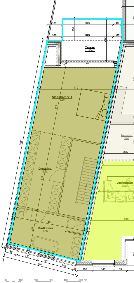
Verdieping 2 - 1/50
