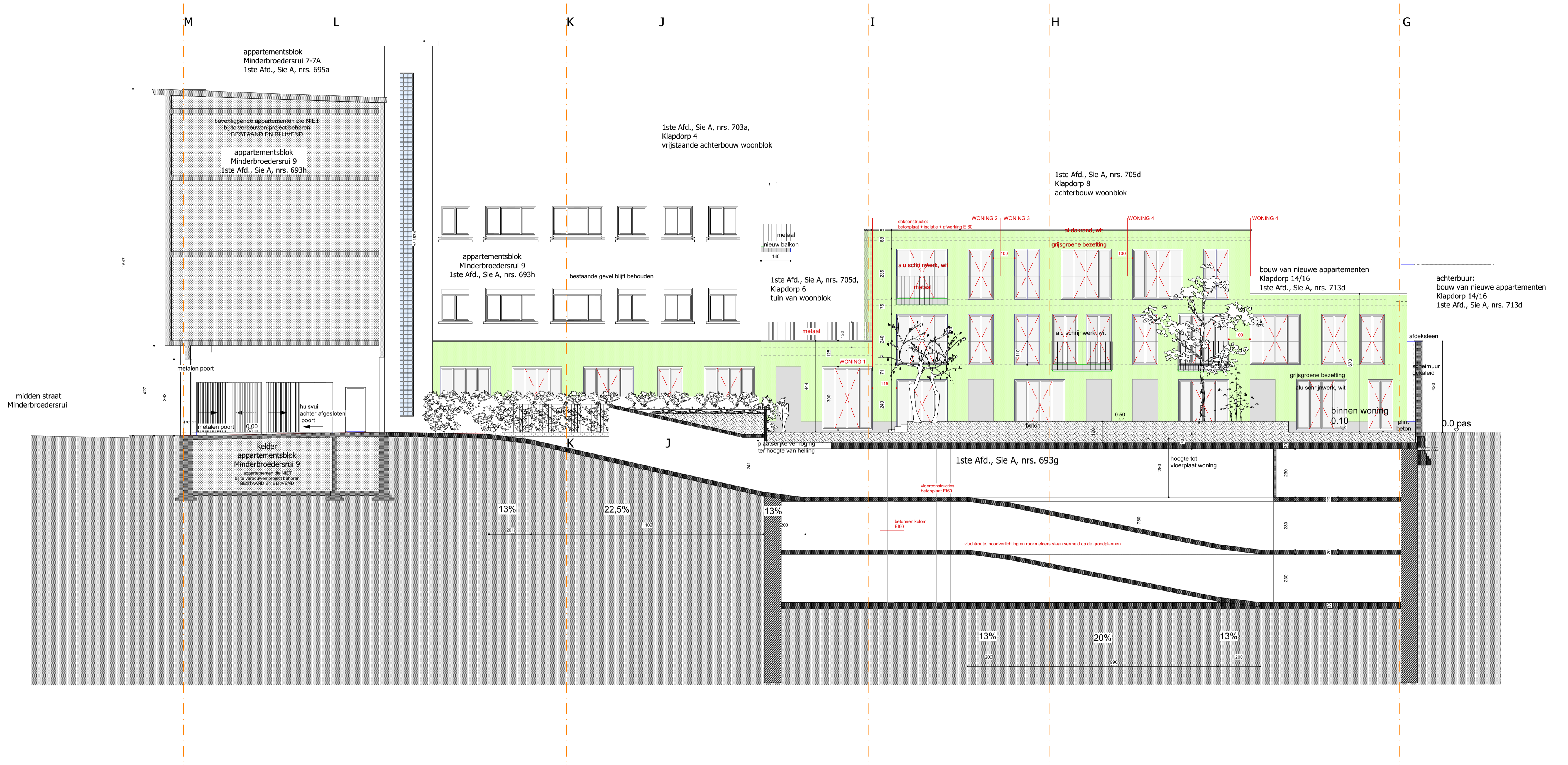
NIEUWE TOESTAND, SNEDE BB' en VOORGEVEL
