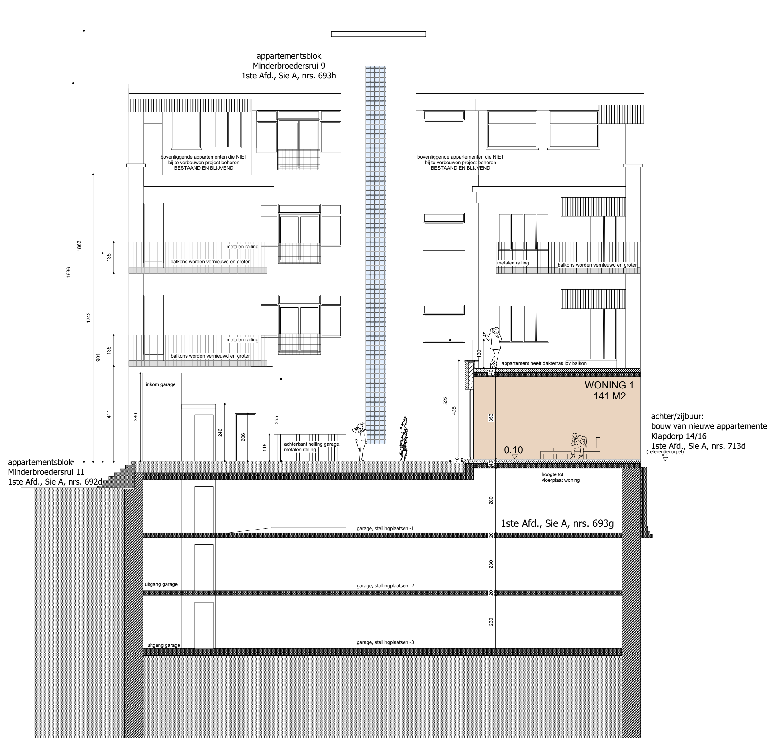
NIEUWE TOESTAND, SNEDE DD'
