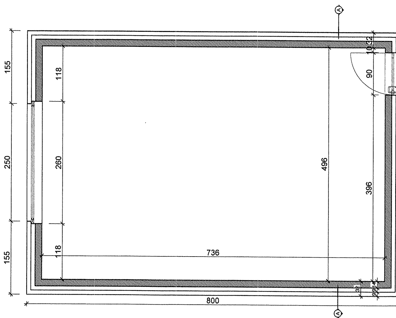
Vue en plan garage
